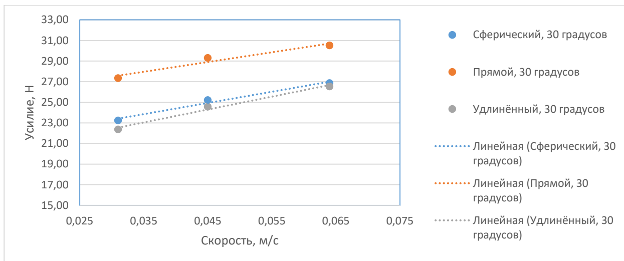
Рисунок 3.8 – Зависимость усилия в вытяжном конце при угле наклона 30° (в уравнениях аппроксимации T – усилие во время выборки, v – скорость выборки)
