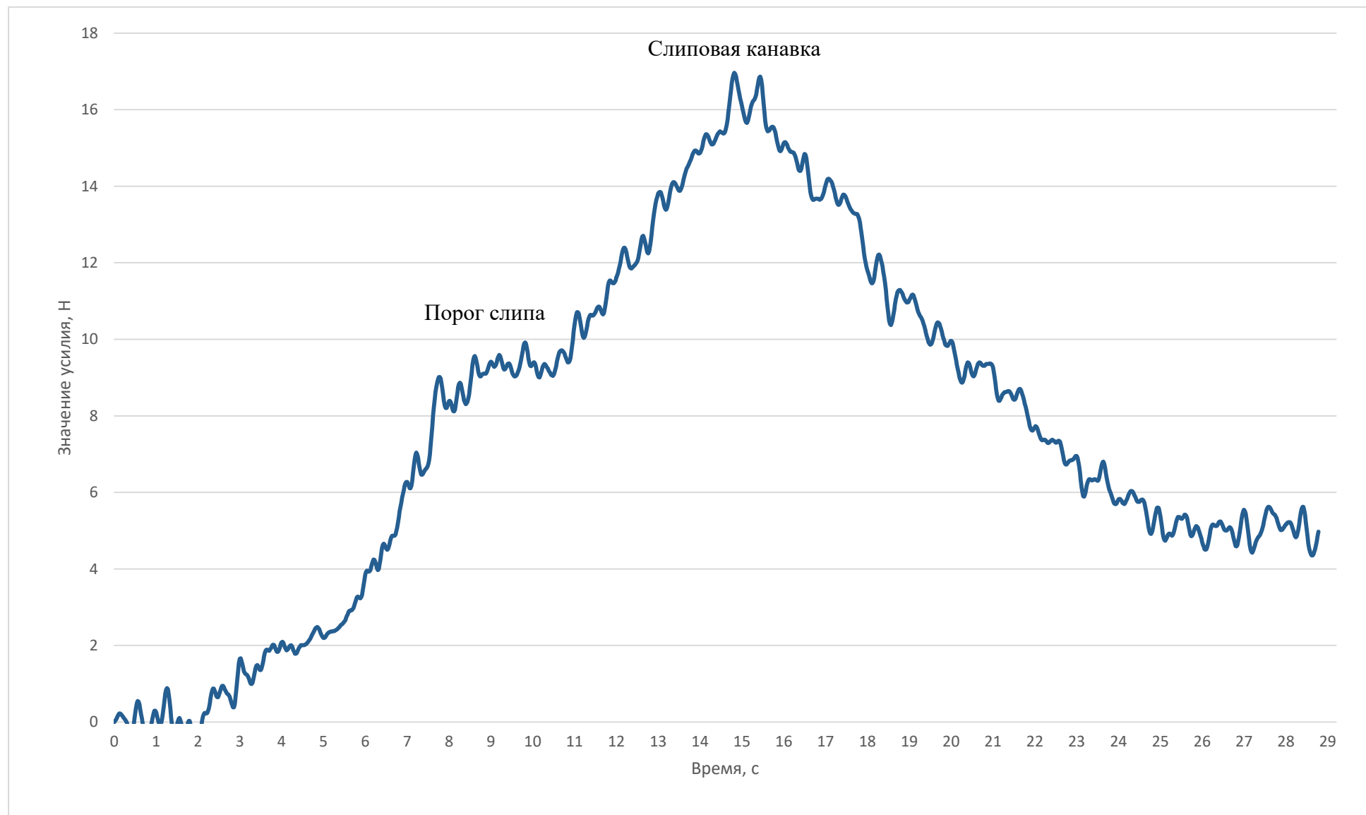
Рисунок П.Б.5 – Динамограмма усилия выборки мешка массой 1,25 кг на макетной установке по слипу сферической формы с углом наклона 30° и угле выхода вытяжного конца 5°
