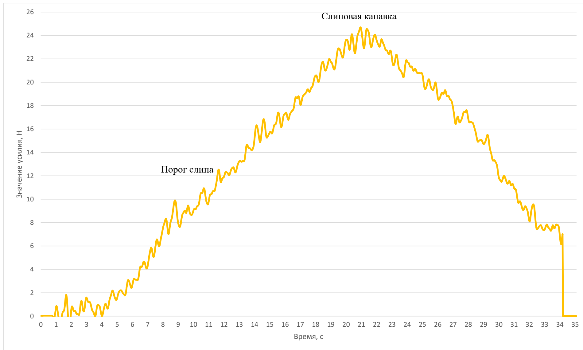
Рисунок П.Б.12 – Динамограмма усилия выборки мешка массой 2,0 кг на макетной установке по слипу прямолинейной формы с углом наклона 45^{\circ} и угле выхода вытяжного конца 20^{\circ}
