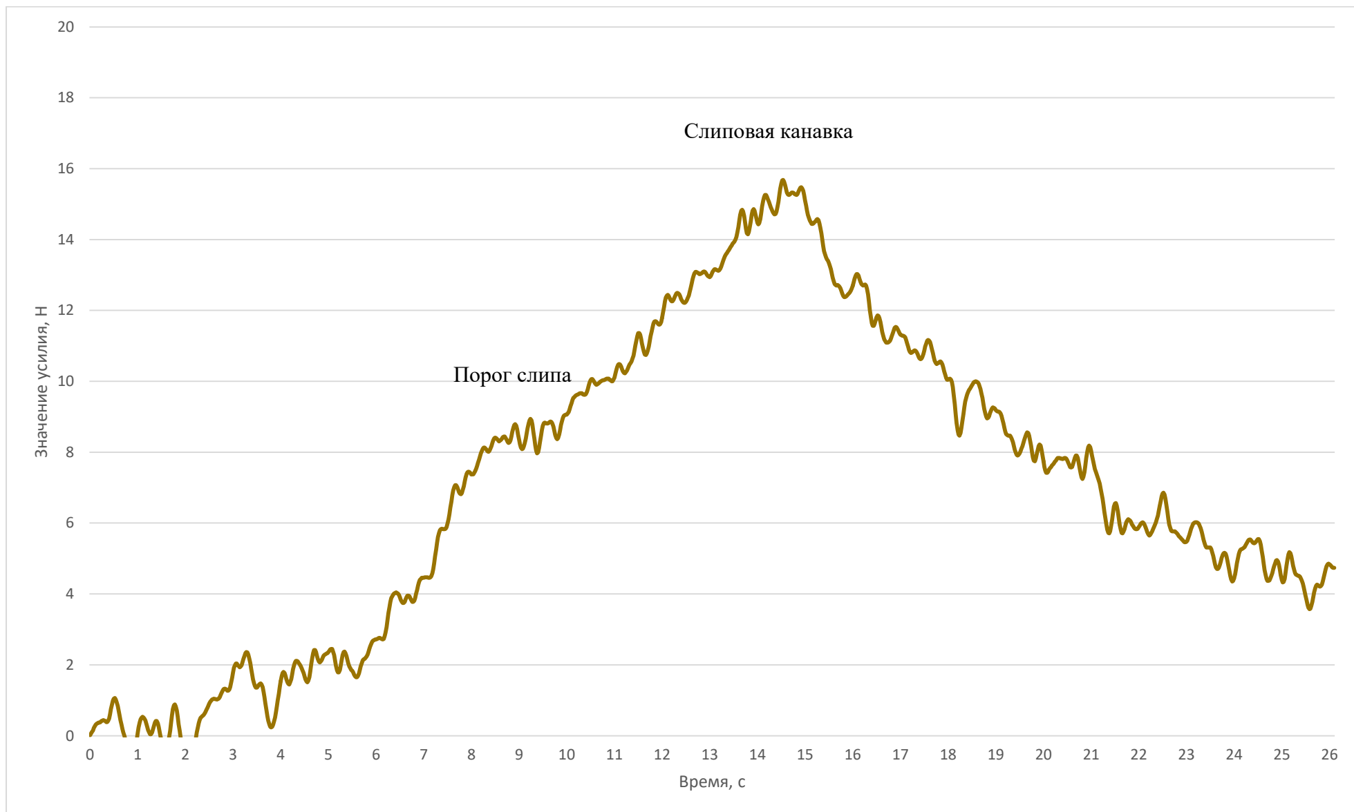
Рисунок П.Б.6 – Динамограмма усилия выборки мешка массой 1,25 кг на макетной установке по слипу сферической формы с углом наклона 30^\circ и угле выхода вытяжного конца 20^\circ
