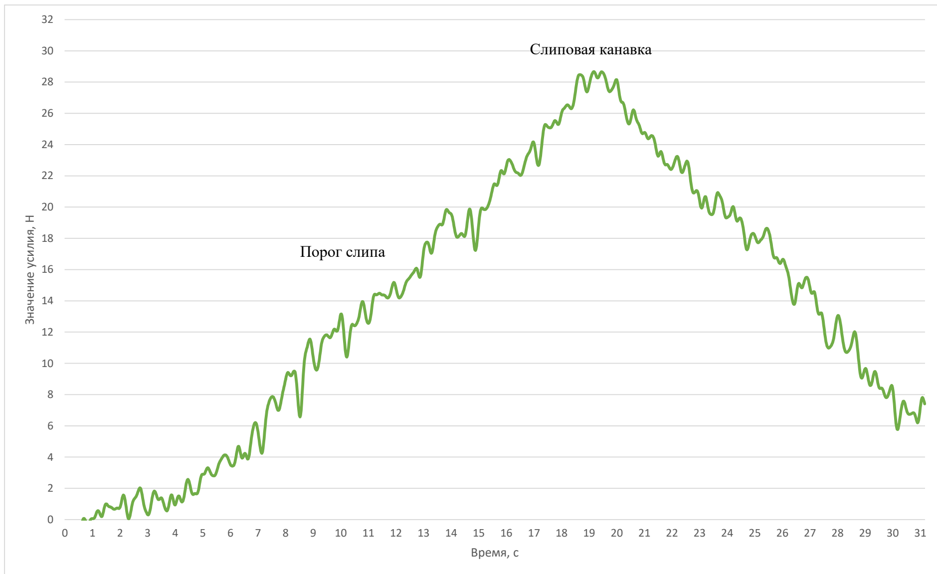
Рисунок П.Б.11 – Динамограмма усилия выборки мешка массой 2,0 кг на макетной установке по слипу прямолинейной формы с углом наклона 45° и угле выхода вытяжного конца 5°
