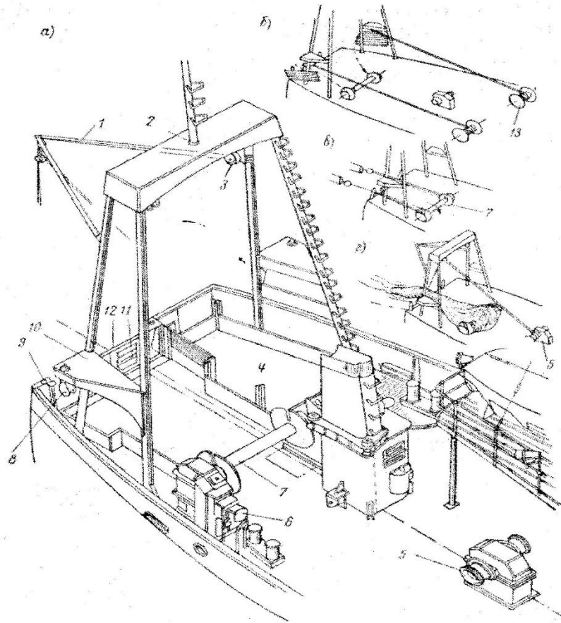
Рисунок 1.14 – Промысловое устройство английского траулера Росс Дэринг:
