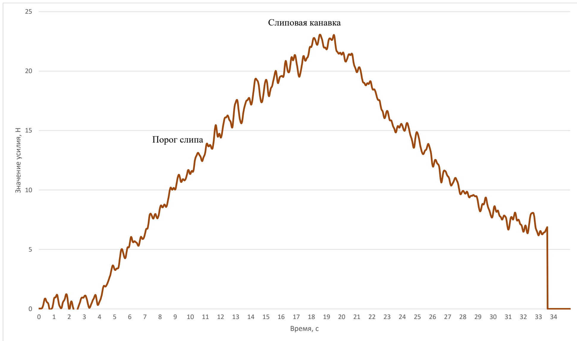
Рисунок П.Б.4 – Динамограмма усилия выборки мешка массой 2,0 кг на макетной установке по слипу сферической формы с углом наклона 45° и угле выхода вытяжного конца 20°
