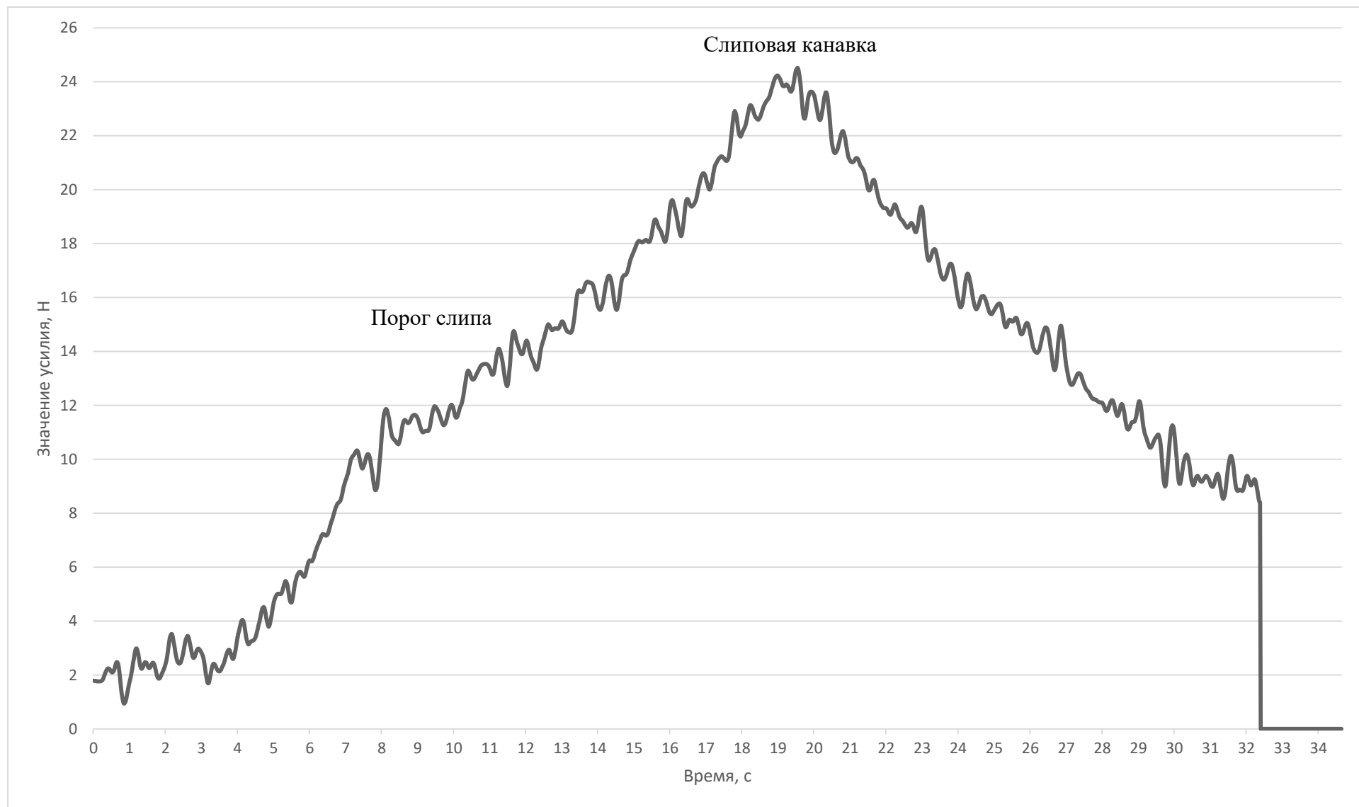
Рисунок П.Б.9 – Динамограмма усилия выборки мешка массой 2,0 кг на макетной установке по слипу прямолинейной формы с углом наклона 30^\circ и угле выхода вытяжного конца 5^\circ
