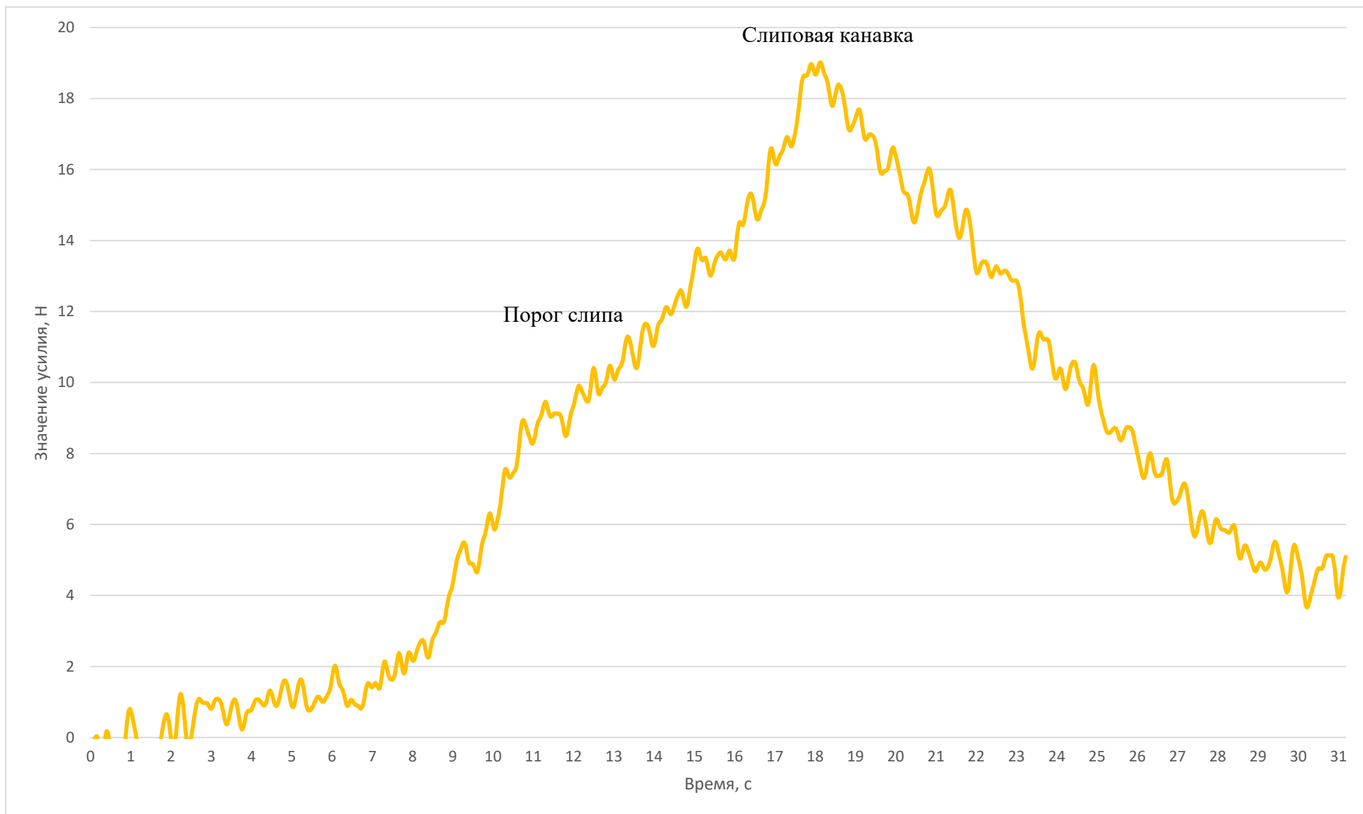
Рисунок П.Б.7 – Динамограмма усилия выборки мешка массой 1,25 кг на макетной установке по слипу сферической формы с углом наклона 45^\circ и угле выхода вытяжного конца 5^\circ
