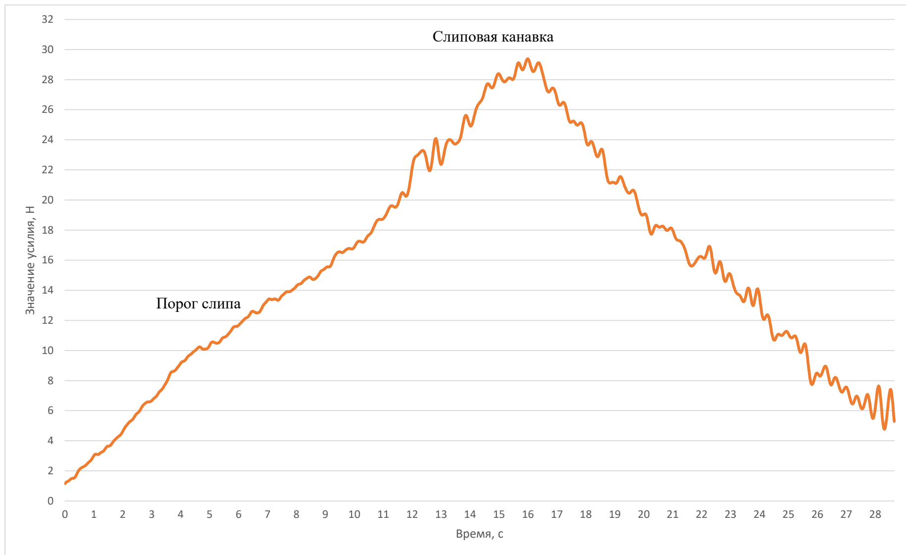
Рисунок П.В.8 – Динамограмма усилия выборки мешка на макетной установке по слипу прямолинейной формы с углом наклона 30^\circ и скоростью выборки 0,048 м/с
