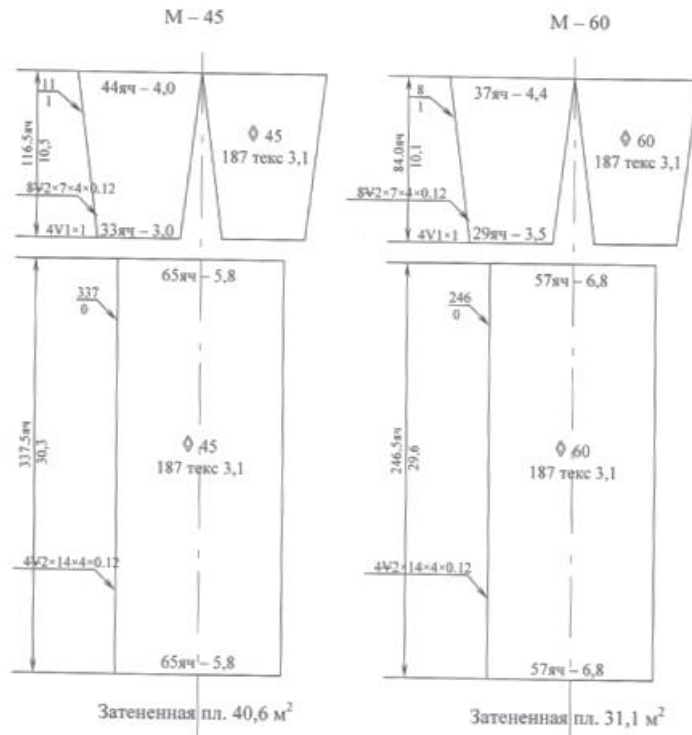
Рисунок 4.4 – Чертёж мешков трала 70/300 М-45 и М-60
