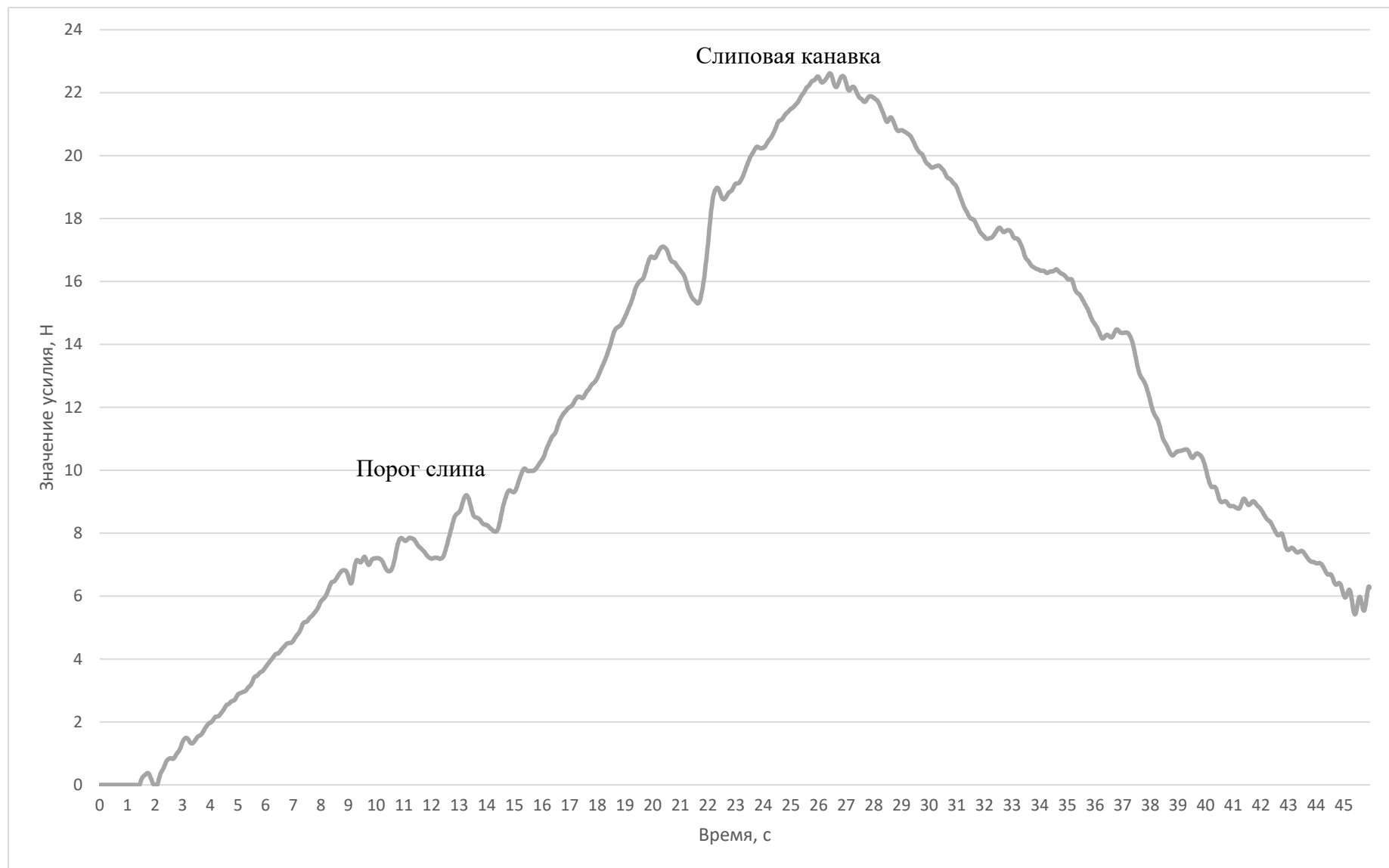
Рисунок П.В.18 – Динамограмма усилия выборки мешка на макетной установке по слипу удлиненной формы с углом наклона 30^\circ и скоростью выборки 0,031 \text{ м/с}
