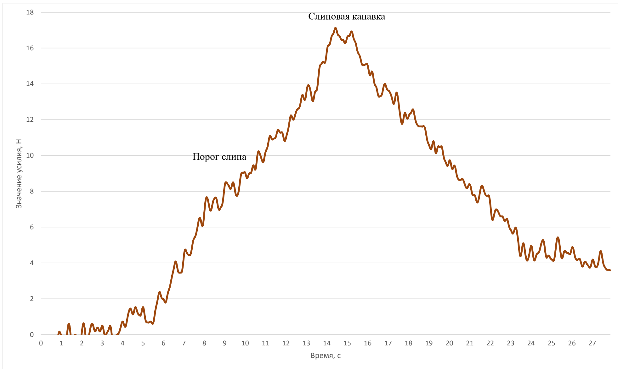
Рисунок П.Б.8 – Динамограмма усилия выборки мешка массой 1,25 кг на макетной установке по слипу сферической формы с углом наклона 45^{\circ} и угле выхода вытяжного конца 20^{\circ}
