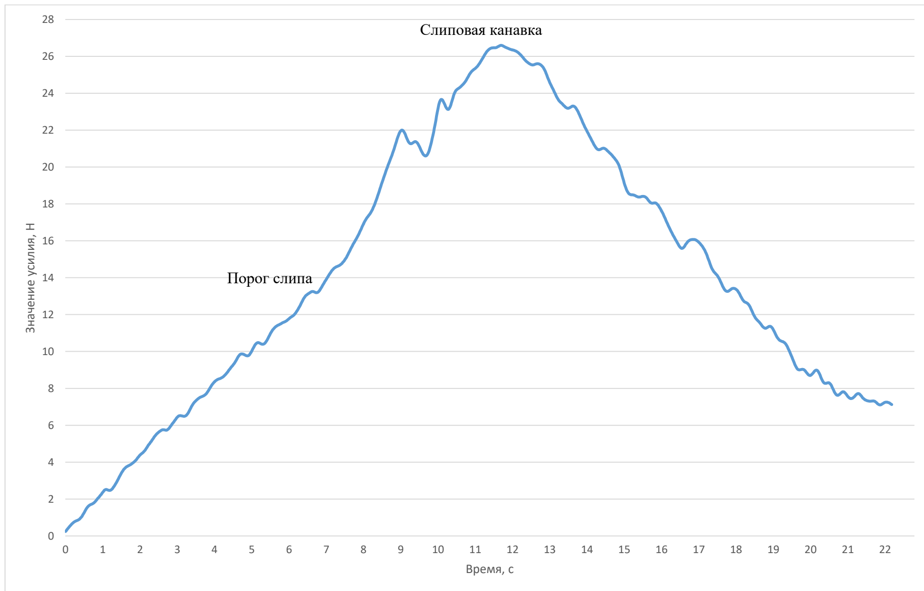
Рисунок П.В.16 – Динамограмма усилия выборки мешка на макетной установке по слипу удлиненной формы с углом наклона 30^\circ и скоростью выборки 0,064 м/с
