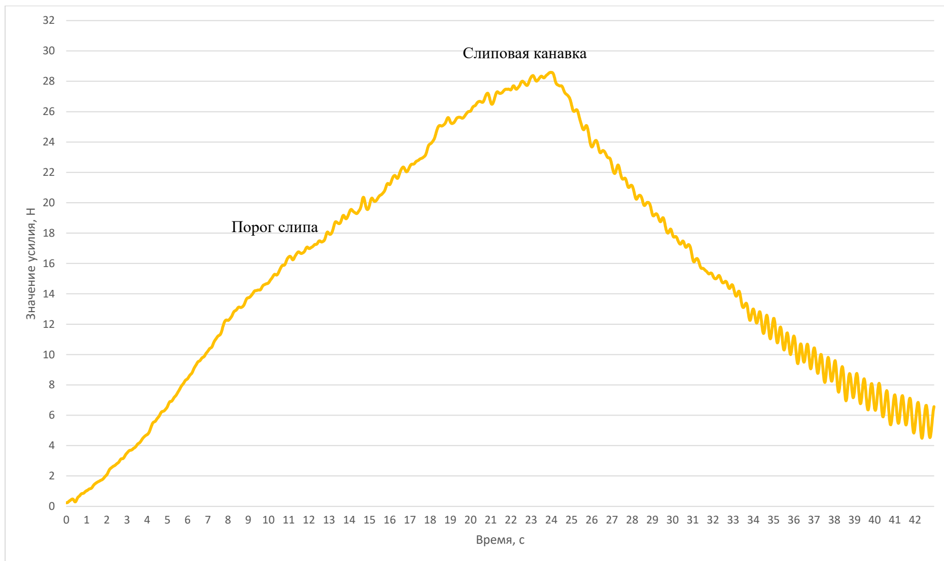
Рисунок П.В.3 – Динамограмма усилия выборки мешка на макетной установке по слипу сферической формы с углом наклона 45^{\circ} и скоростью выборки 0,031 м/с
