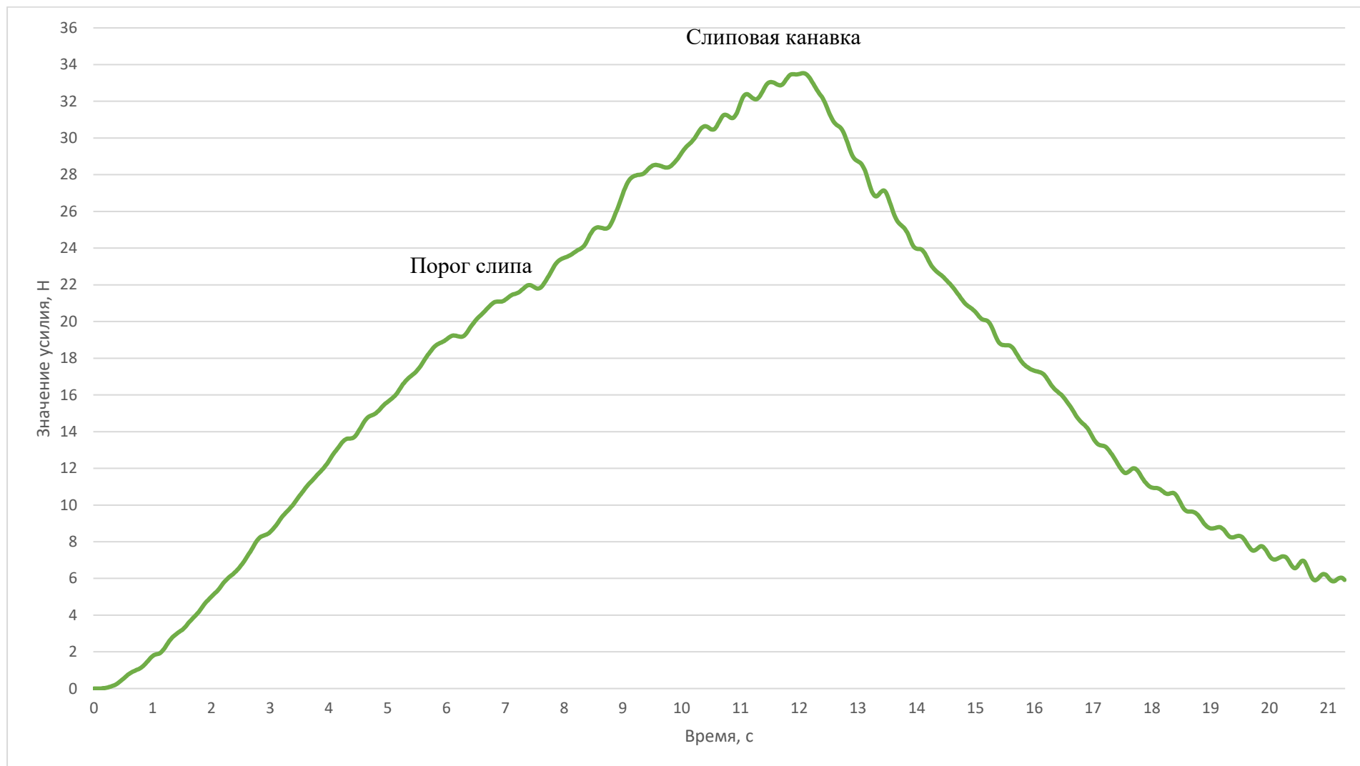
Рисунок П.В.1 – Динамограмма усилия выборки мешка на макетной установке по слипу сферической формы с углом наклона 45^\circ и скоростью выборки 0,064 м/с
