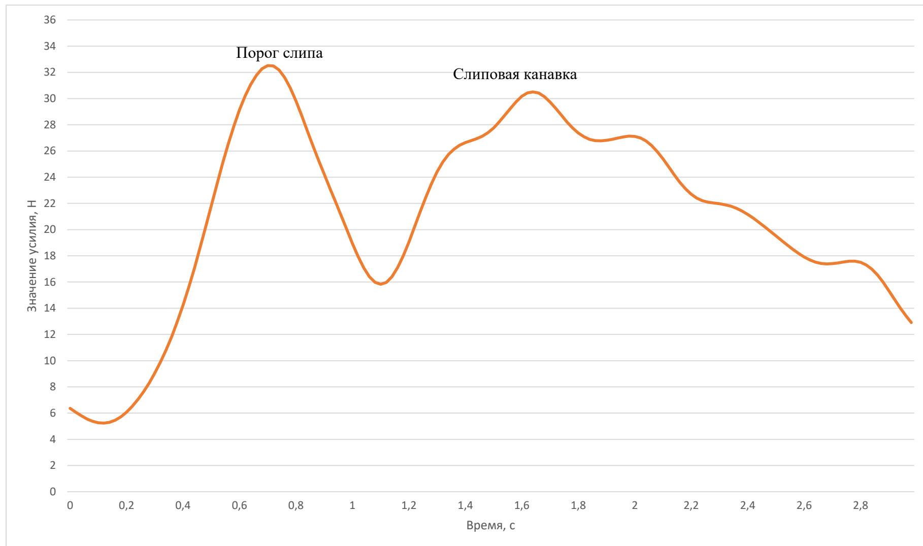
Рисунок П.Г.5 – Динамограмма усилия выборки мешка на макетной установке по слипу прямой формы с углом наклона 30^\circ , скоростью выборки 0,4 м/с и площадью соприкосновения мешка и слипковой поверхности 246 \text{ см}^2
