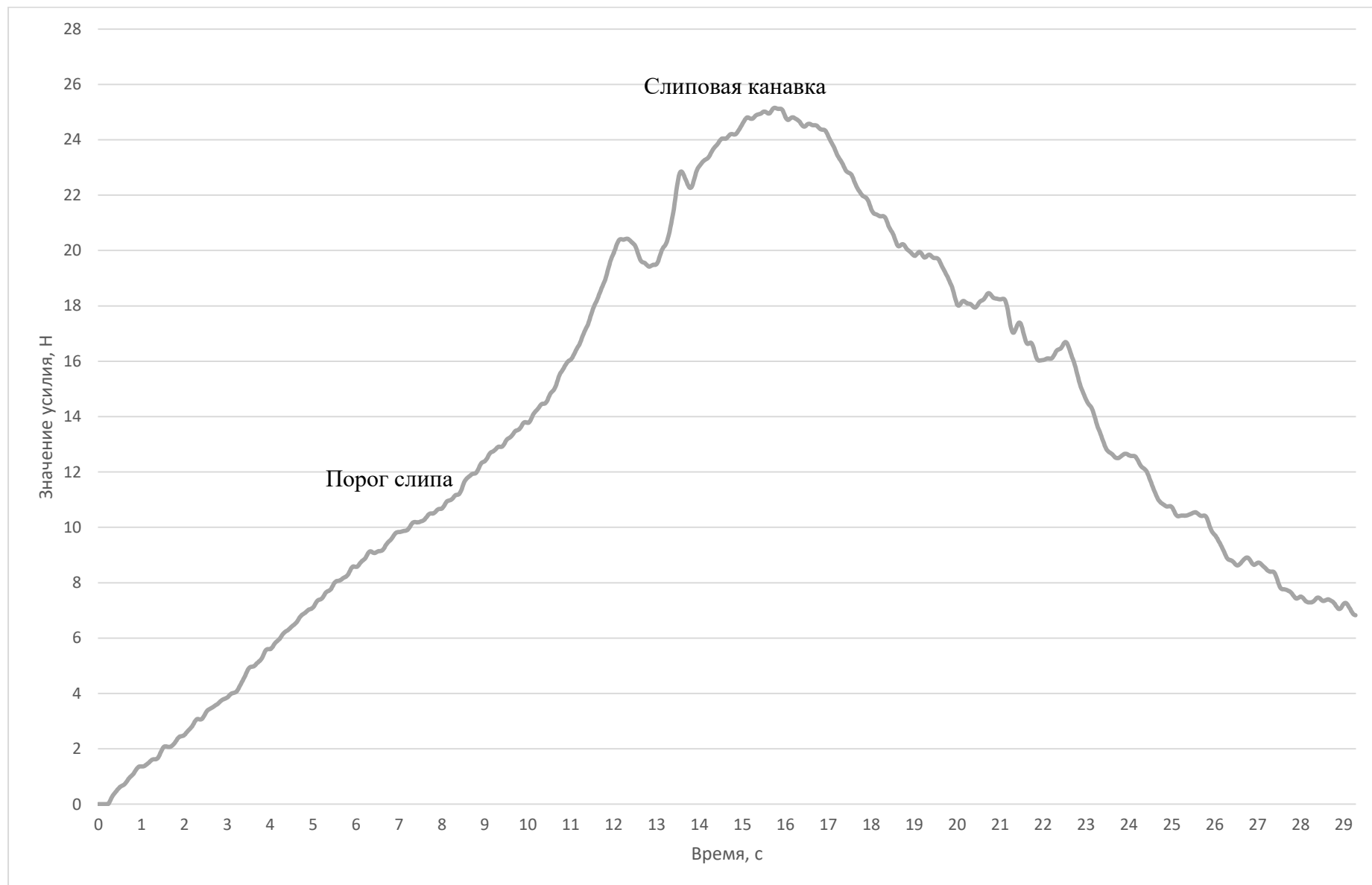
Рисунок П.В.17 – Динамограмма усилия выборки мешка на макетной установке по слипу удлинённой формы с углом наклона 30^\circ и скоростью выборки 0,048 \text{ м/с}
