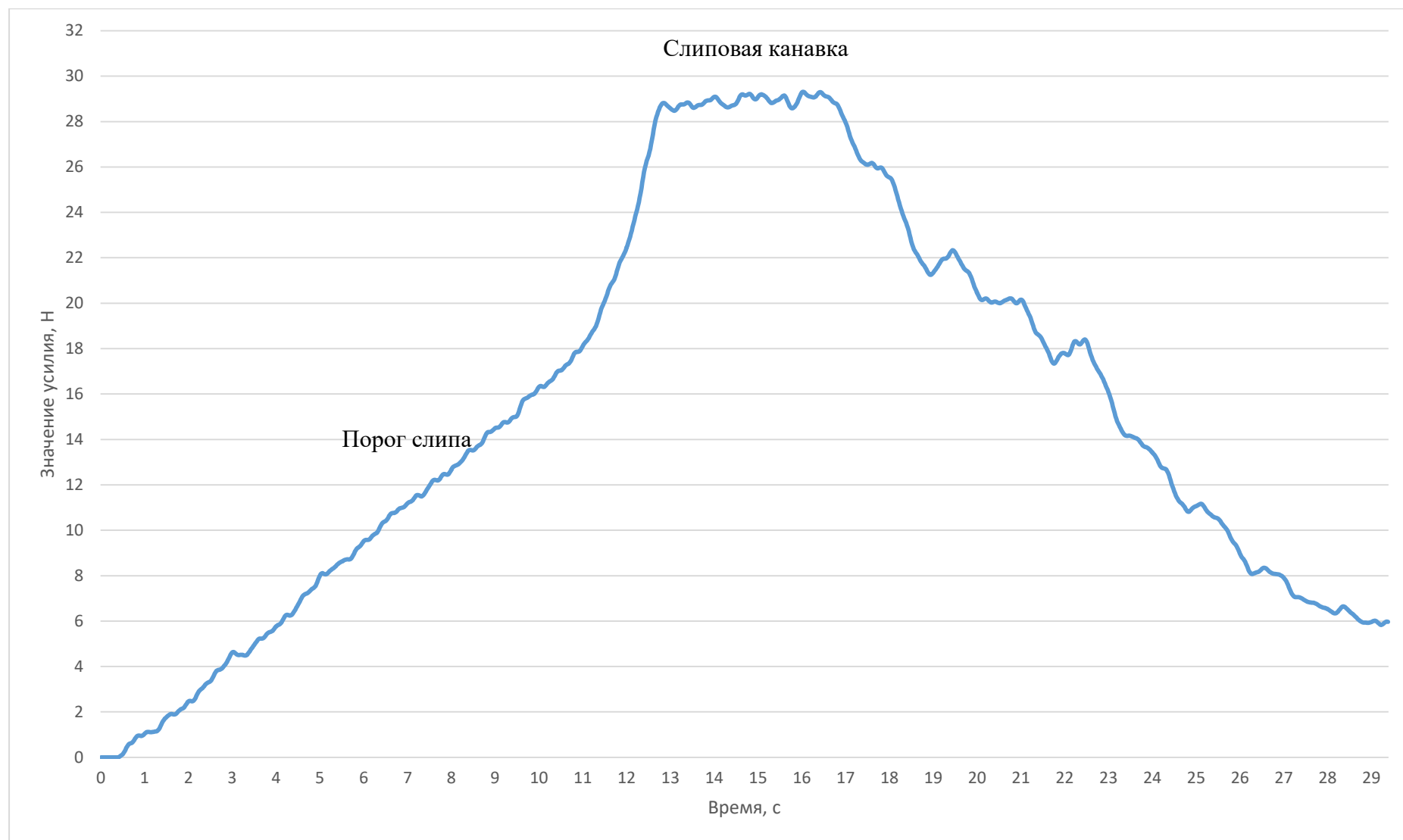
Рисунок П.В.14 – Динамограмма усилия выборки мешка на макетной установке по слипу удлинённой формы с углом наклона 45^\circ и скоростью выборки 0,048 м/с
