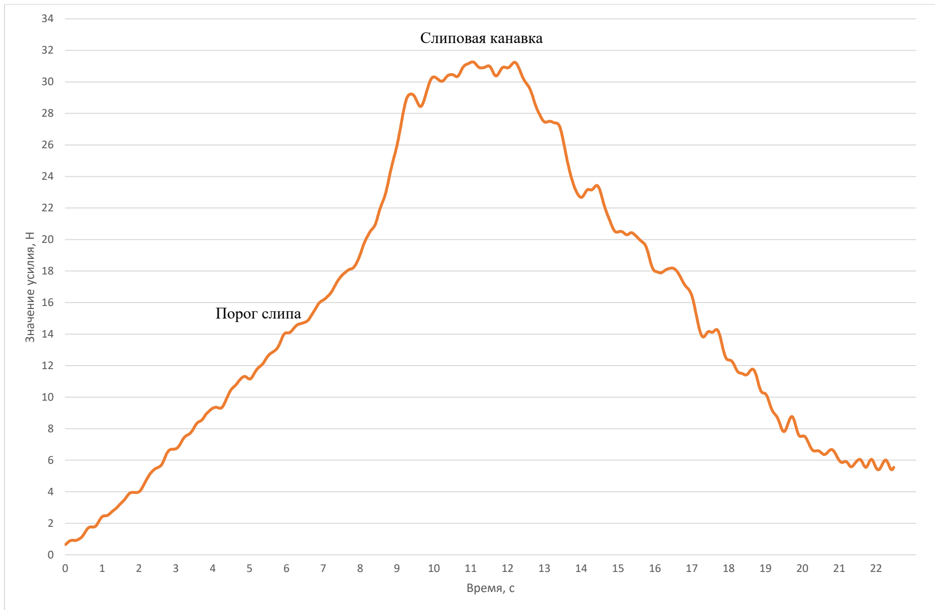
Рисунок П.В.13 – Динамограмма усилия выборки мешка на макетной установке по слипу удлинённой формы с углом наклона 45^\circ и скоростью выборки 0,064 м/с
