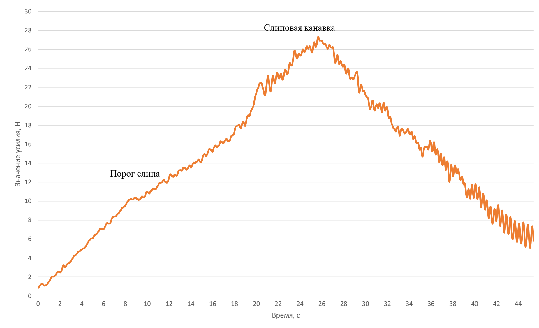
Рисунок П.В.7 – Динамограмма усилия выборки мешка на макетной установке по слипу прямолинейной формы с углом наклона 30^\circ и скоростью выборки 0,031 \text{ м/с}
