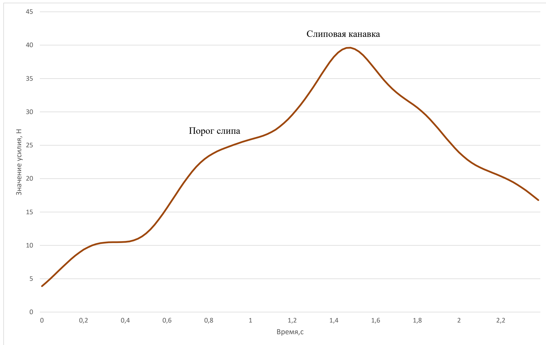
Рисунок П.Г.11 – Динамограмма усилия выборки мешка на макетной установке по слипу сферической формы с углом наклона 45^\circ , скоростью выборки 0,5 м/с и площадью соприкосновения мешка и слипковой поверхности 246 \text{ см}^2
