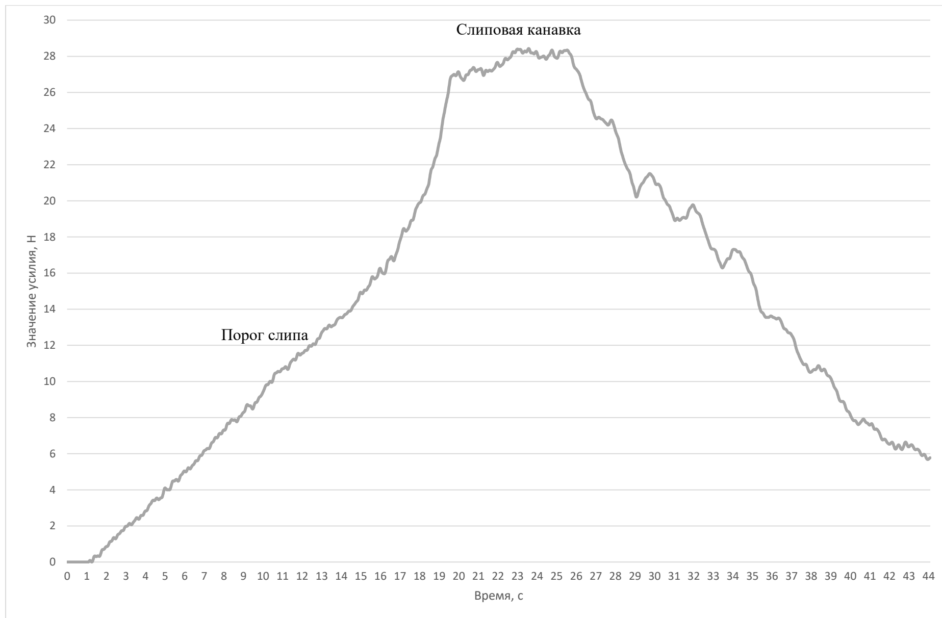
Рисунок П.В.15 – Динамограмма усилия выборки мешка на макетной установке по слипу удлиненной формы с углом наклона 45^\circ и скоростью выборки 0,031 \text{ м/с}
