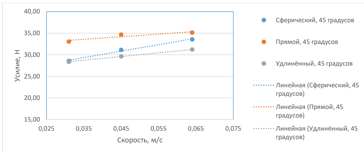
Рисунок 3.9 – Зависимость усилия в вытяжном конце при угле наклона 45 ° (в уравнениях аппроксимации T – усилие во время выборки, v – скорость выборки)
