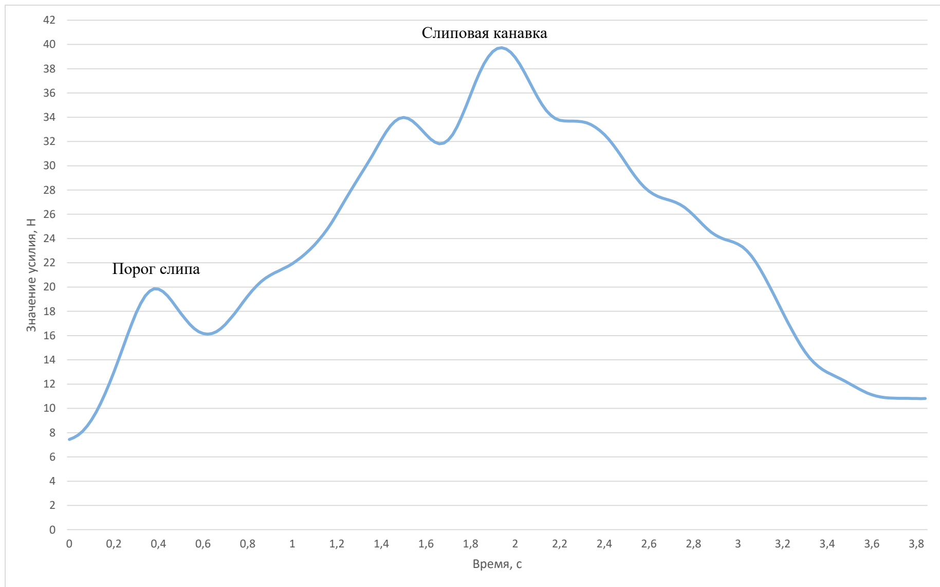
Рисунок П.Г.2 – Динамограмма усилия выборки мешка на макетной установке по слипу прямой формы с углом наклона 45^\circ , скоростью выборки 0,3 м/с и площадью соприкосновения мешка и слипсовой поверхности 246 \text{ см}^2
