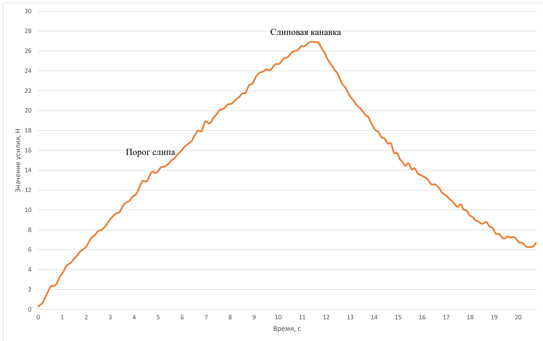
Рисунок П.В.4 – Динамограмма усилия выборки мешка на макетной установке по слипу сферической формы с углом наклона 30^{\circ} и скоростью выборки 0,064 м/с
