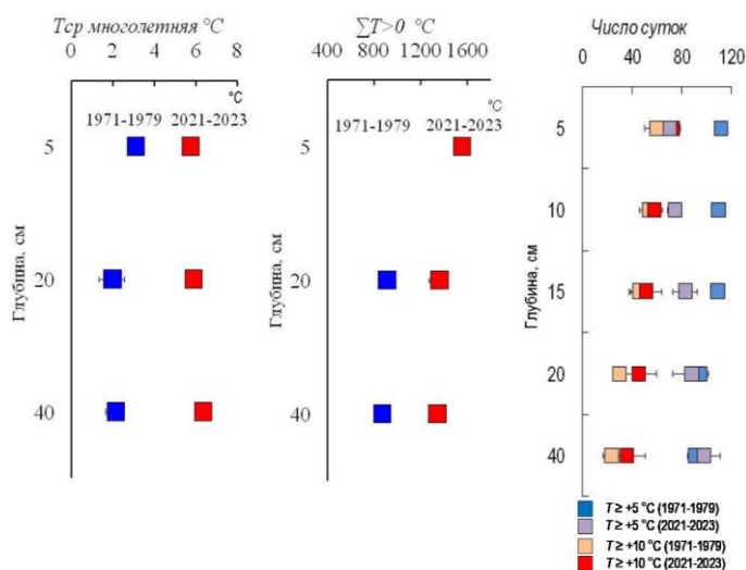
Рисунок 8 – Среднемноголетние значения годовой температуры в профиле зонального лесного подзола на предгорной равнине в 1971–1979 и 2021–2023 гг.
