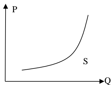
Рисунок 6 – Кривая предложения
