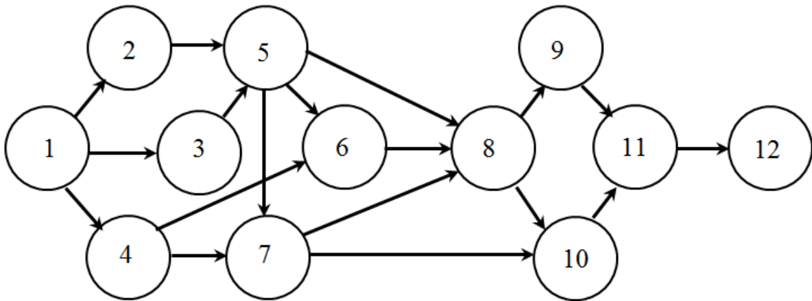
Рис. 10.5.1. Сетевая модель организации морской грузовой линии.
