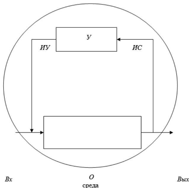
Рис. 1.1.1. Схема управления с обратной связью У – управляющая система; О – объект управления; ИУ – канал передачи управляющей информации; ИС – информация о состоянии (передачи информации о состоянии объекта); Вх– вход; Вых – выход.
