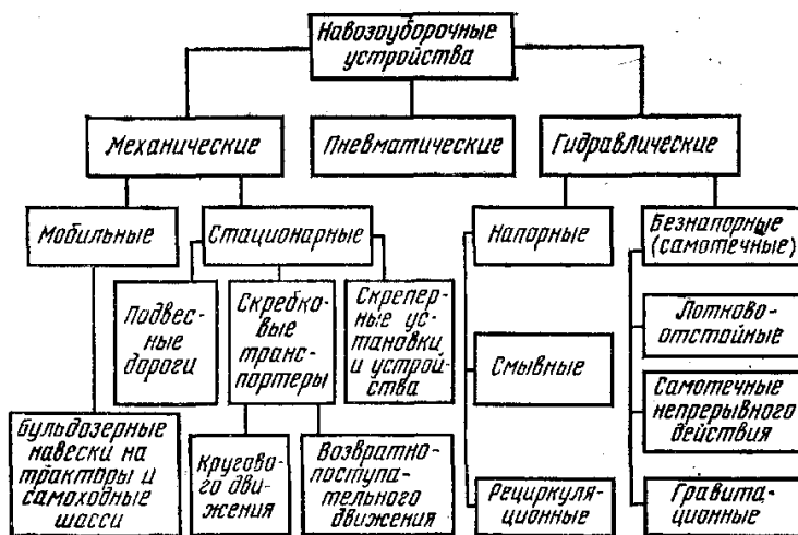
Рисунок 6 – Классификация устройств для удаления навоза из помещений
