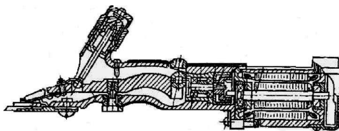
Рисунок 5 – Стригальная машинка МСУ-200
