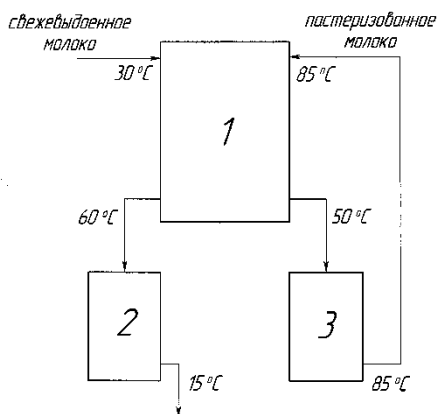
Рисунок 3 – Схема включения проточного регенератора в молочную линию: 1 – регенератор; 2 – охладитель; 3 – пастеризатор
