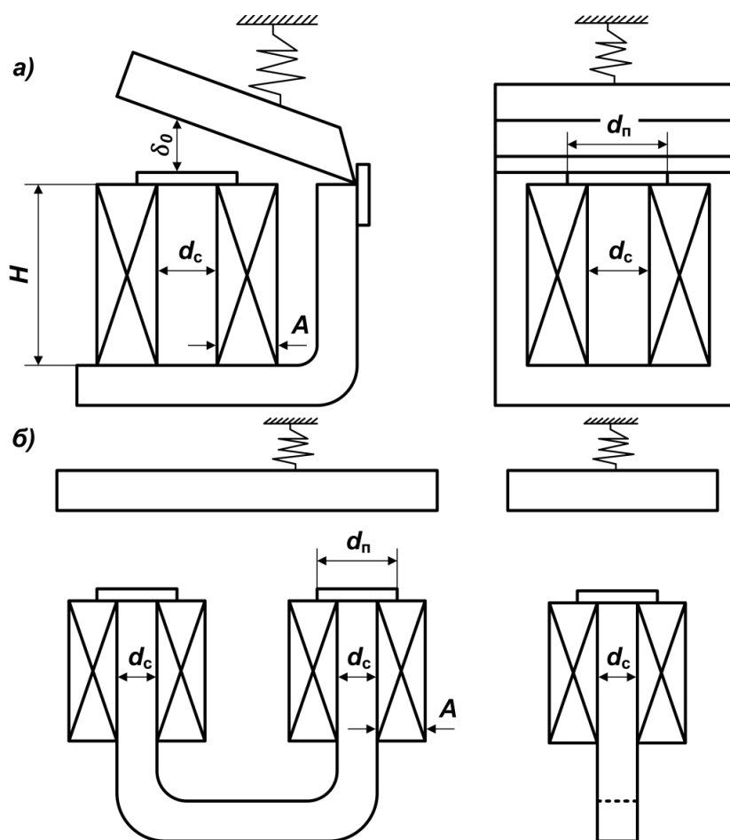
Рисунок 2.1 – Эскизы электромагнитов: поворотного (а); прямоходовой (б)
