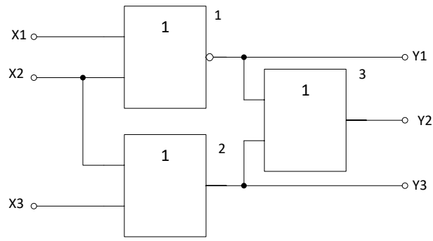
Рисунок 7 – Схема диагностируемого объекта
