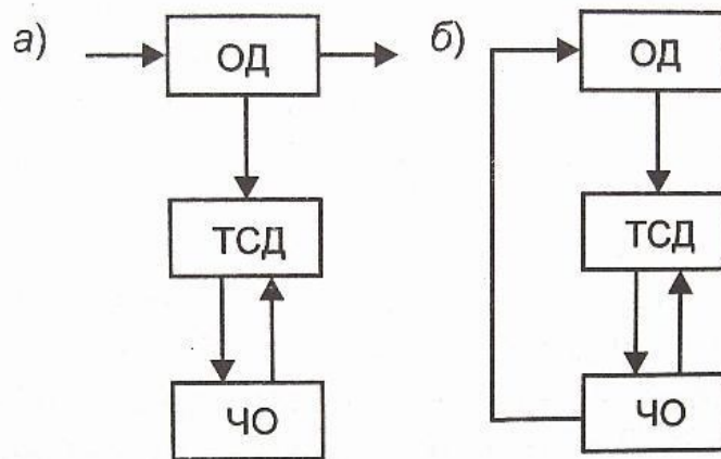
Рисунок 3 - Структурные схемы рабочего диагностирования
