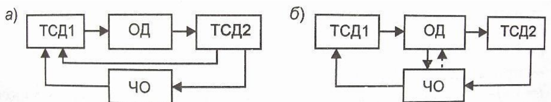
Рисунок 4 - Структурные схемы тестового диагностирования:
