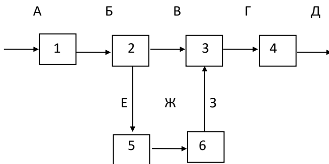
Рисунок 6 - Функциональная схема электропривода вентилятора
