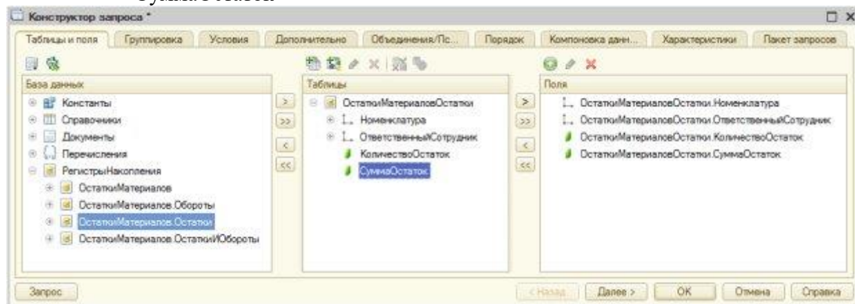
Рисунок 9.18. Создание запроса
