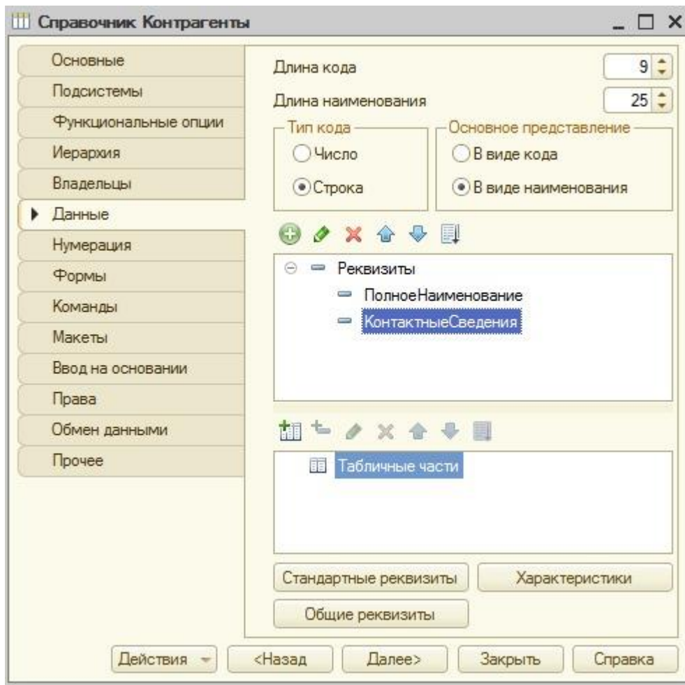
Рисунок 7.12. Справочник Контрагенты
