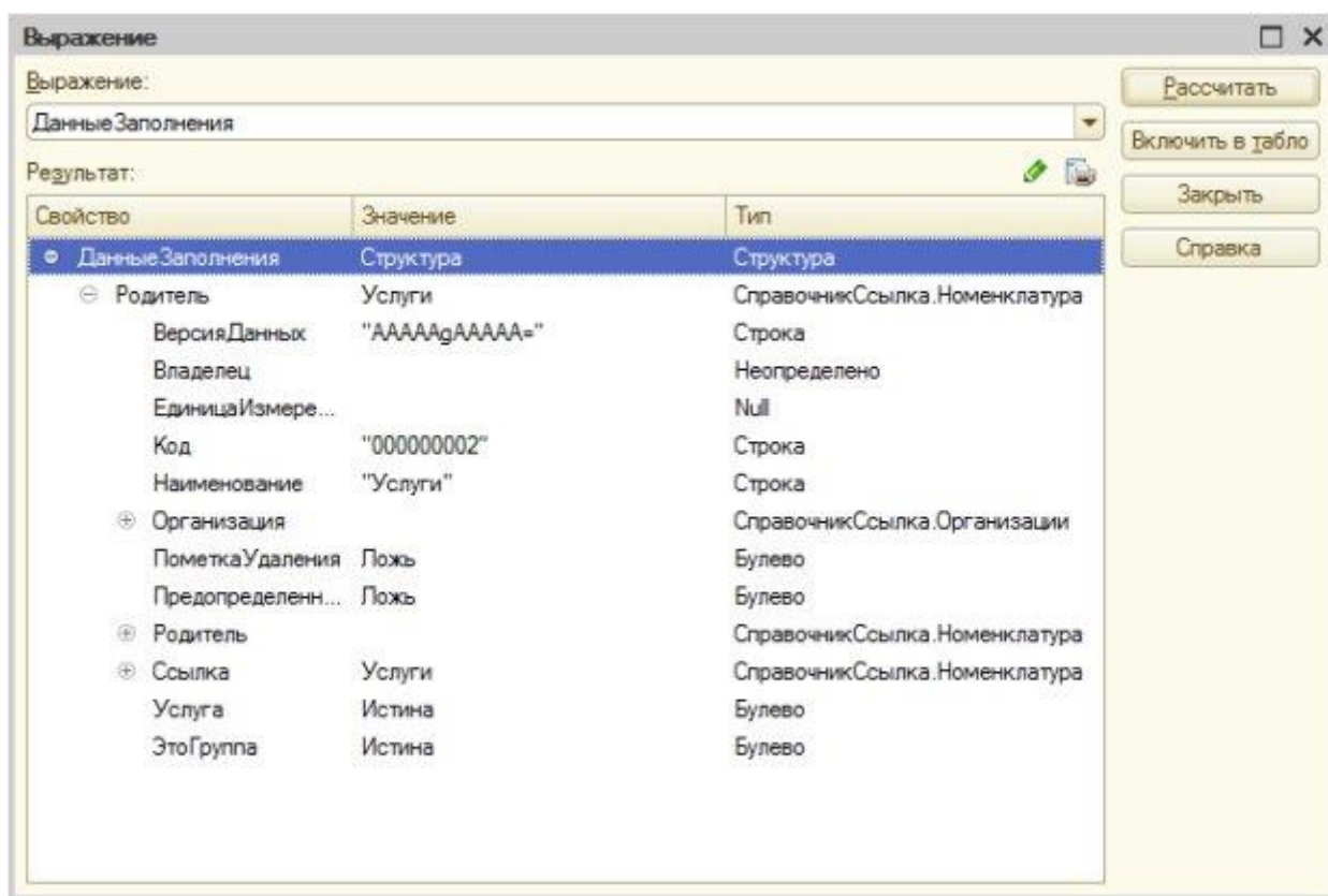
Рисунок 7.6. Структура ДанныеЗаполнения
