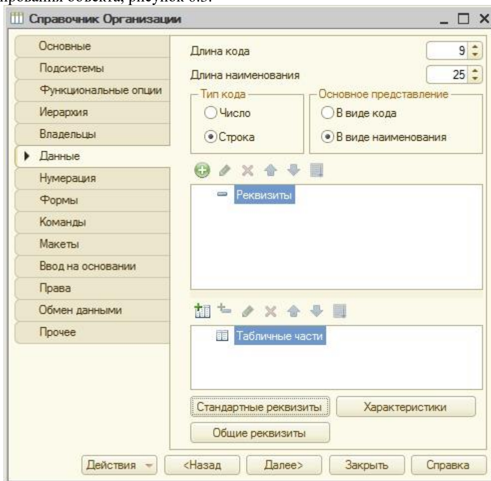
Рисунок 6.3. Настройка справочника
