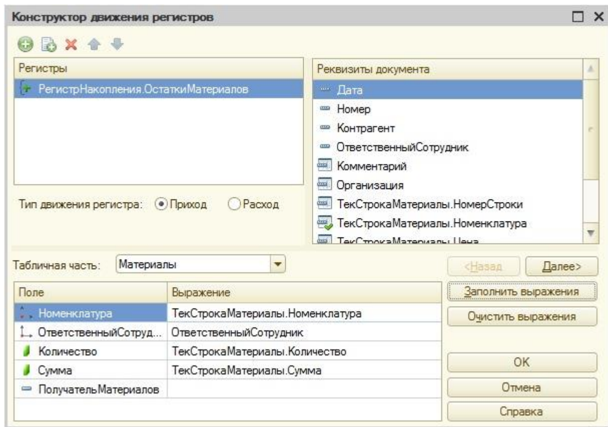
Рисунок 9.15. Конструктор движений
