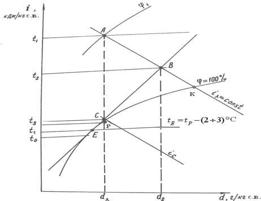
Рисунок 4 – Цикл работы ТНСУ в i - d -диаграмме влажного воздуха
