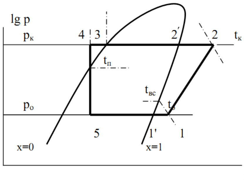
Рисунок 2 – Рабочий цикл одноступенчатого хладонового теплового насоса с регенеративным теплообменником
