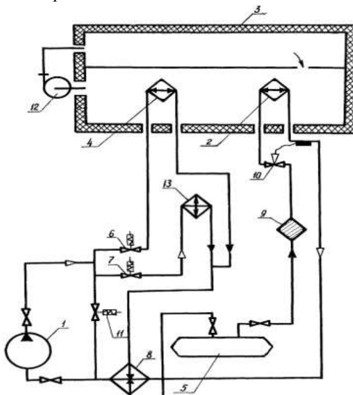
Рисунок 3 – Схема ТНСУ для вяления и сушки рыбы:
