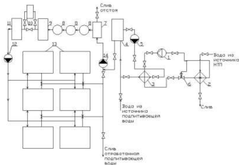
Рисунок 5 – Схема установки замкнутого обеспечения для разведения рыб с теплонасосной установкой (ТНУ) с одним компрессором для термоподготовки воды 1 – компрессор ТНУ; 2 – испаритель ТНУ; 3 – конденсатор ТНУ; 4 – бак-аккумулятор; 5 – насос водяной; 6 – регулирующий вентиль ТНУ; 7 – механический фильтр; 8 – биофильтр; 9 – бактерицидная лампа; 10 – оксигенатор; 11 – расходная емкость; 12 – насос водяной; 13 – рыбоводные бассейны; 14 – насос водяной
