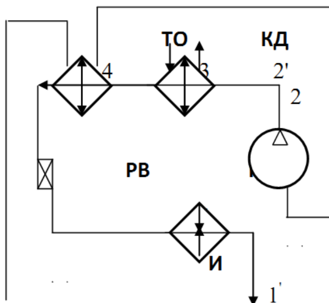
Рисунок 1 – Схема одноступенчатой хладонового теплового насоса с регенеративным теплообменником
