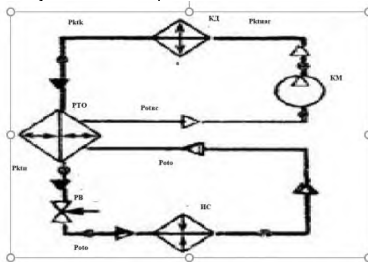
Рисунок 22. Регенеративный теплообменник.
