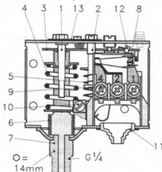
Рисунок 33. Реле давления серии КР.
