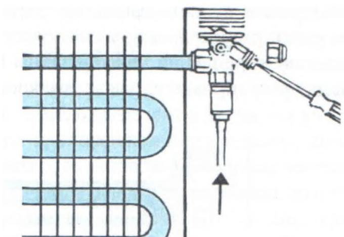
Рисунок 38. Настройка ТРВ. Изменение положения регулировочного винта.
