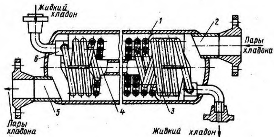
Рисунок 22. Регенеративный теплообменник.
