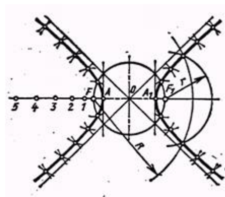
Рисунок 6 Гипербола
