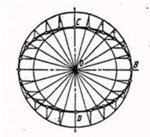
Рисунок 3 Циклоида
