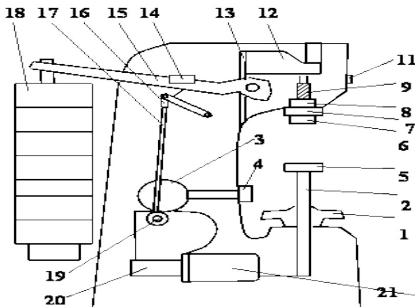
Рис.1. - Схема прибора для определения твердости по Бринеллю
