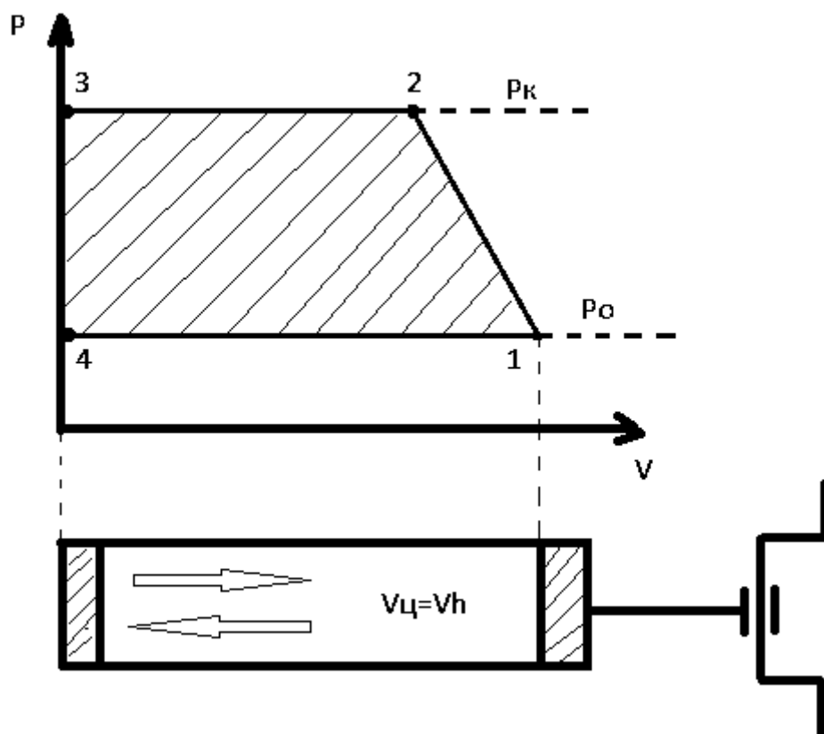
Действительный поршневой компрессор.
