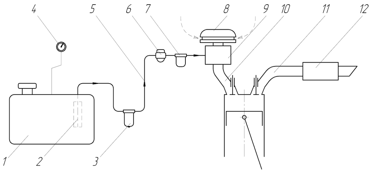
Схема системы питания карбюраторного двигателя
