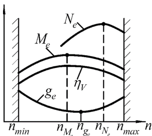
Рис. 1. Внешняя скоростная характеристика
