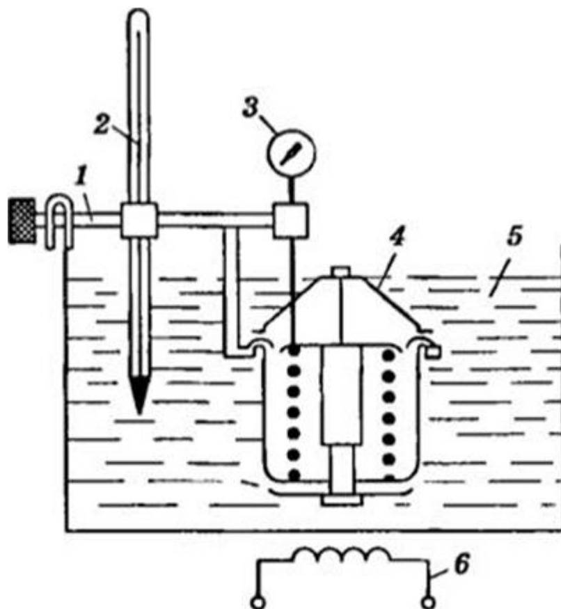
Схема установки для проверки термостата: 1 - кронштейн; 2 - термометр; 3 - индикатор перемещений; 4 - термостат; 5 - ванна с водой; 6 – электронагреватель
