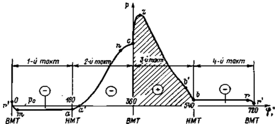
Рис. 2. Развернутая индикаторная диаграмма четырехтактного дизельного двигателя.
