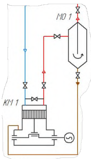
Рисунок 40. Компрессор поршневой и маслоотделитель с перегородкой.
