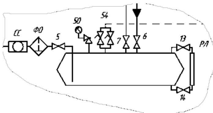
Рисунок 33. Ресивер линейный с фильтром осушителем и смотровым стеклом.
