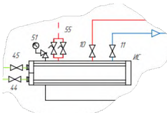
Рисунок 30. Кожухотрубный испаритель без сухопарника.
