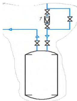
Рисунок 39. Отделитель жидкости
