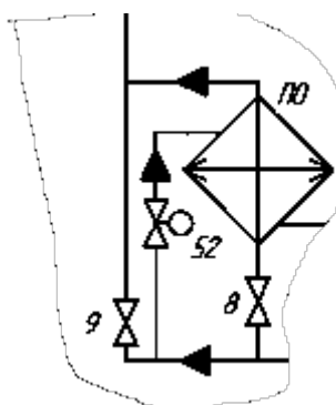
Рисунок 31. Переохладитель (экономайзер).
