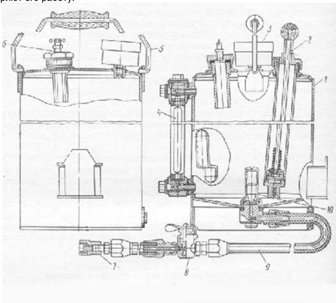
Переносной прибор для проверки герметичности системы питания НИИАТ-383:
