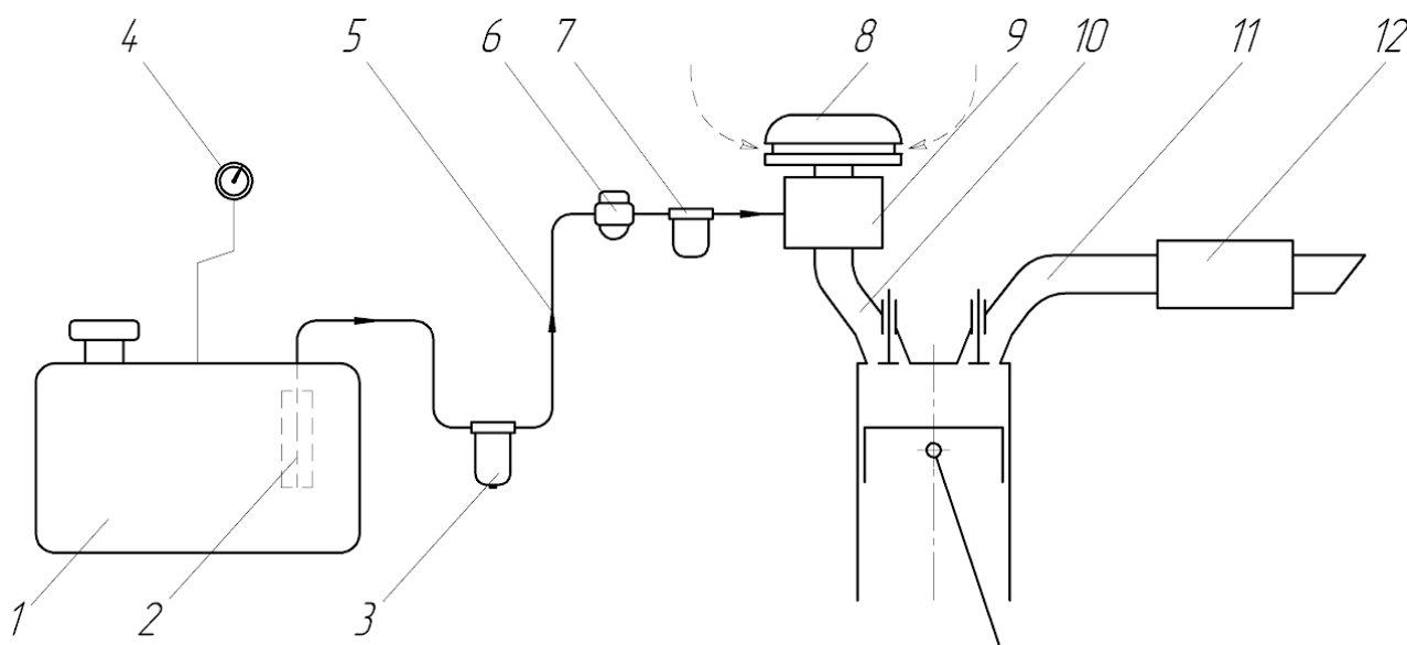
Схема системы питания карбюраторного двигателя
