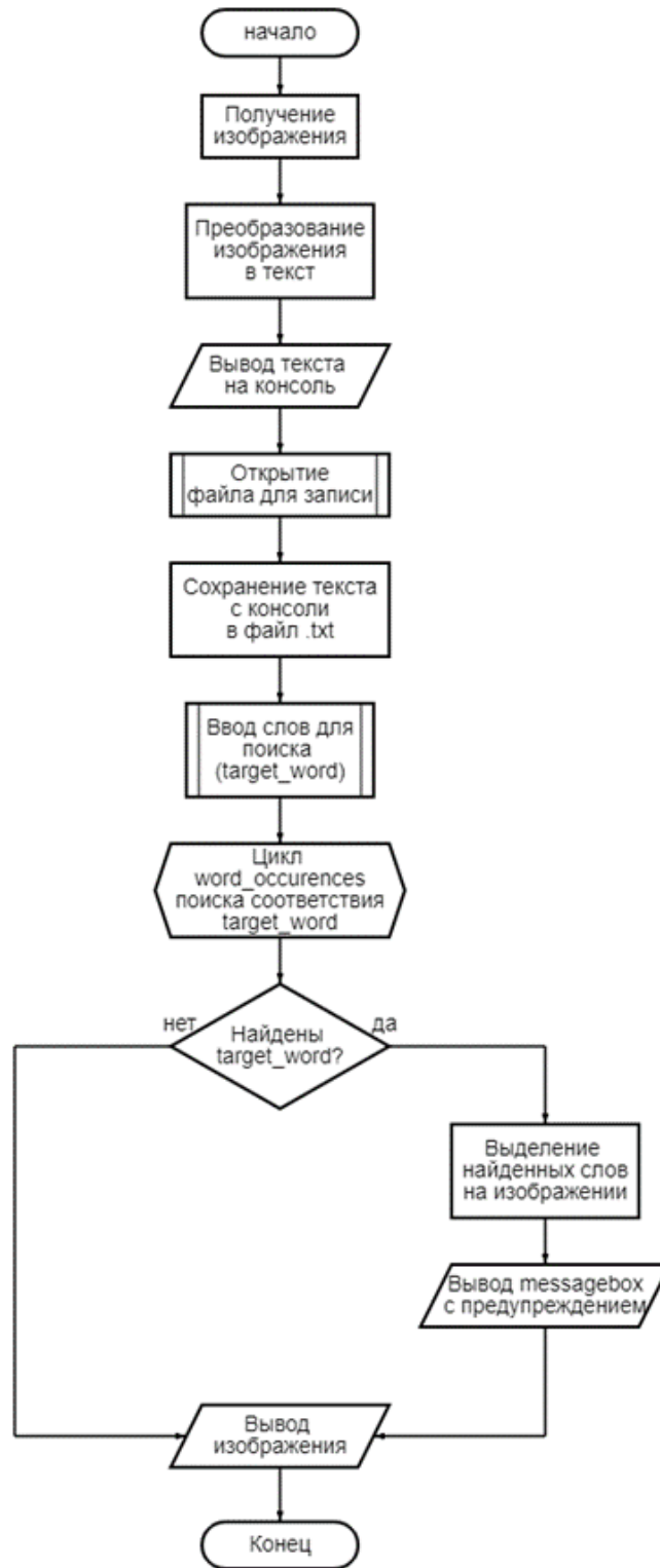
Рисунок 1 – Блок-схема программы
