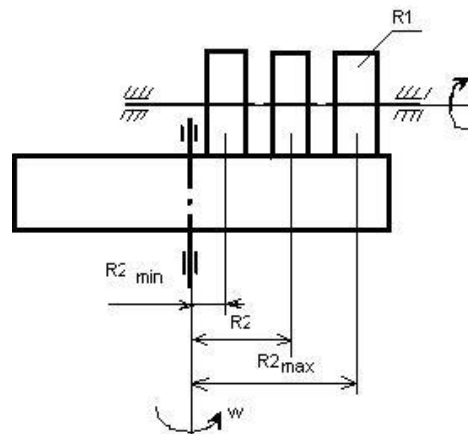
Рисунок 1 Лобовой вариатор
