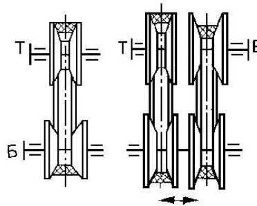
Рисунок 2. Вариаторы с раздвижными конусами
