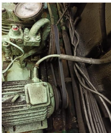
Рисунок 59. Фотография привода с ремнем.
