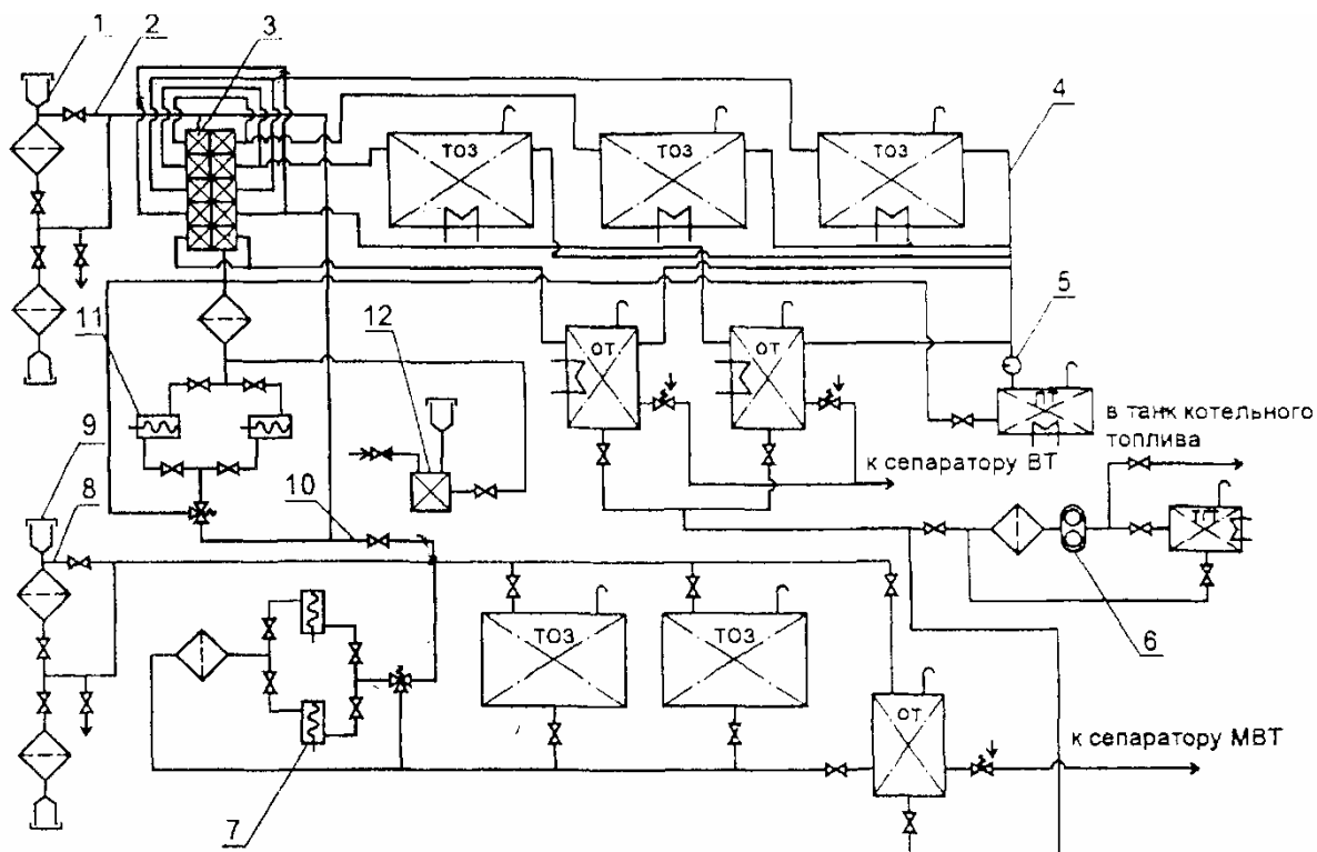
Рисунок 1 – Схема участка приема, хранения, перекачивания МВТ и ВТ.
