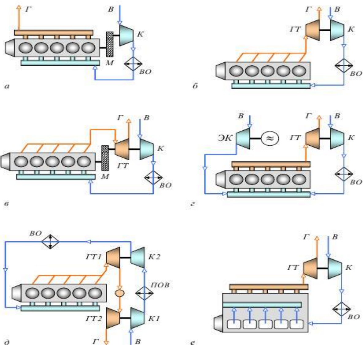
Схемы надува 4-х тактных ДВС
