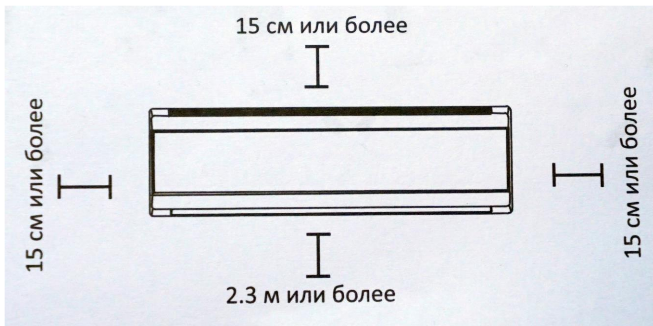
Рис. 2 Рекомендуемые монтажные расстояния
