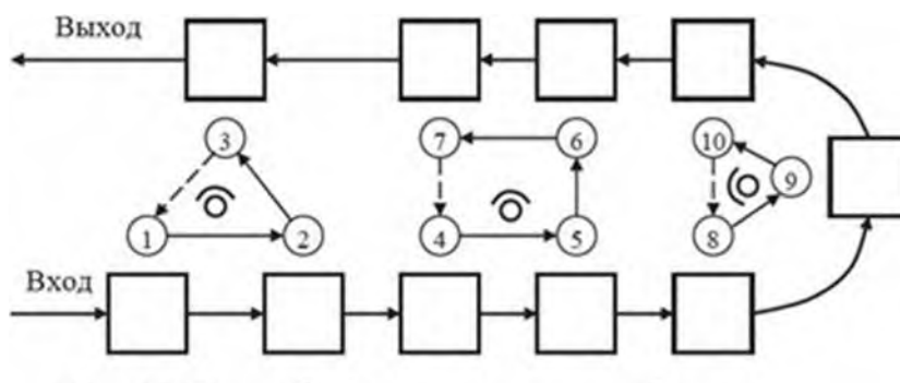
Рисунок 1 – Пример U-образного размещения оборудования
