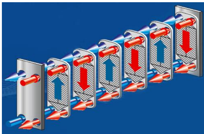
Рисунок 9. Пластинчатый теплообменник. Группа 1.
