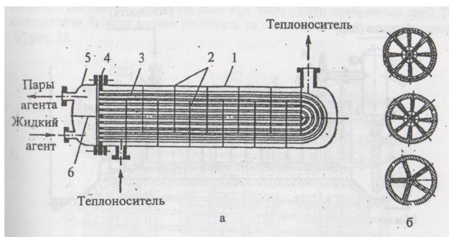
Рисунок 8. Кожухомеевиковый с внутритрубным кипением. Группа 1.
