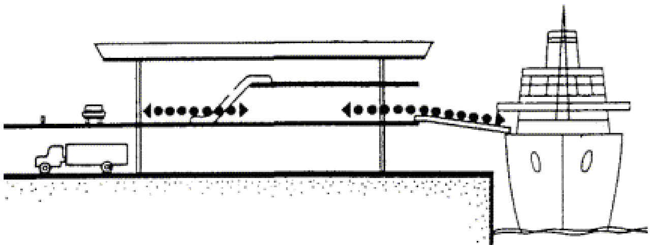
Рисунок - Вариант разделения уровней пассажирских и грузовых операций
