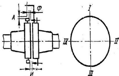
Рисунок 2. Схема замера зазоров для определения соосности центрируемых валов. А-радиальный зазор. Ф,И- осевые зазоры.
