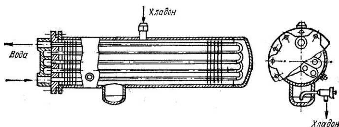
Рисунок 4. Кожухотрубный конденсатор. Группа 1.
