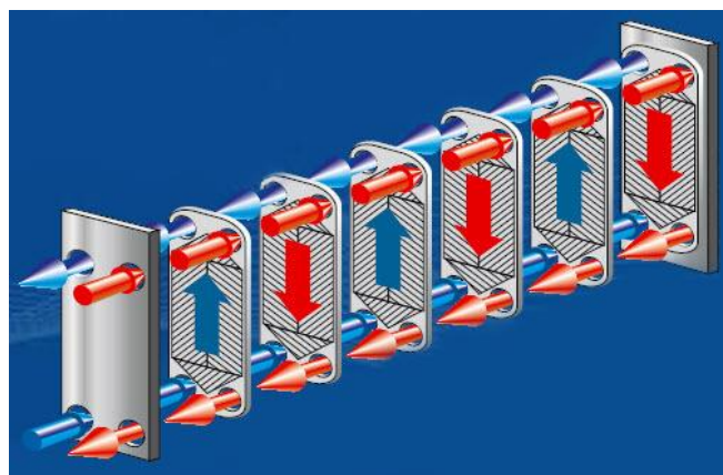
Рисунок 9. Пластина́тный теплообменник. Группа 1.
