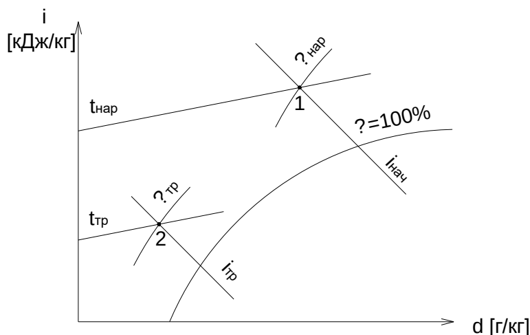
Рис. 4.1 Диаграмма влажного воздуха.
