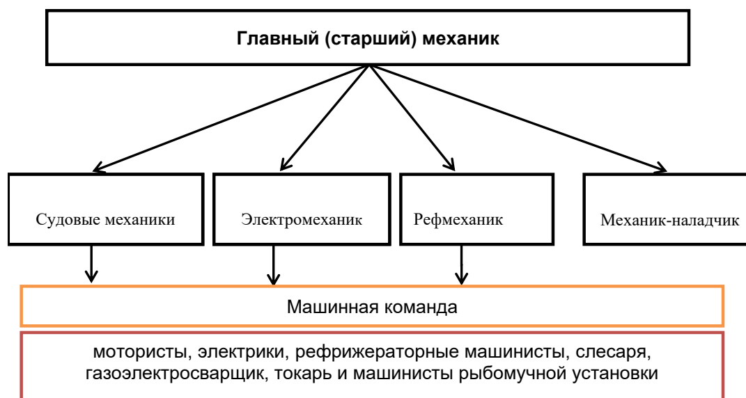
Рис.1 Функциональная схема судомеханической службы рыбодобывающего судна.
