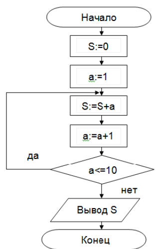
Рис. Циклический алгоритм с постусловием
