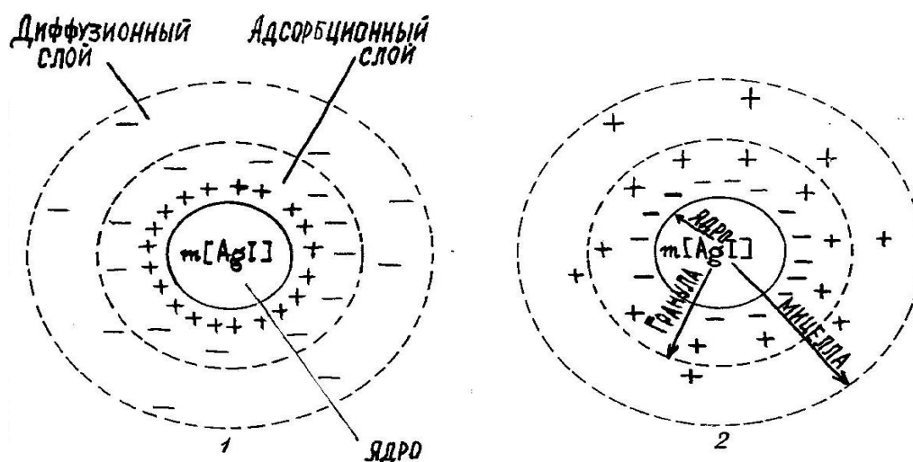
Рисунок 1 – Строение мицелл золя йодистого серебра, полученного в избытке AgNO_3 (I) и KI (II)
