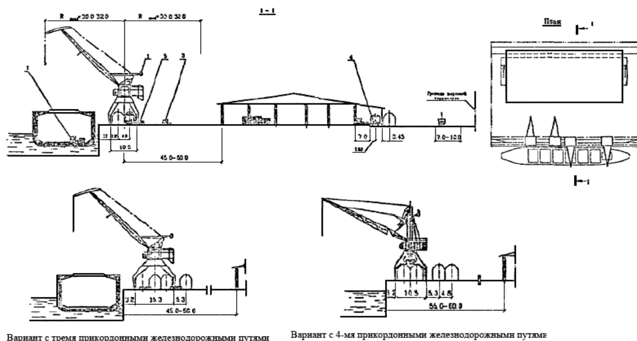
Рисунок – Примеры схем технологического процесса
