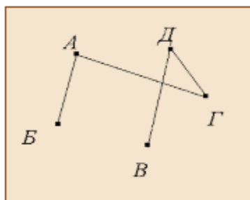
Рис. 3 Неполный граф
