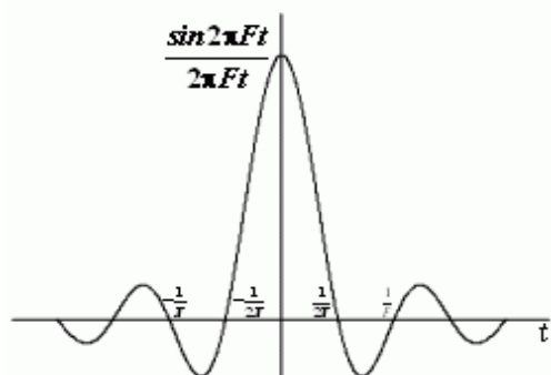
Рис. 1.17. Функция отсчётов
