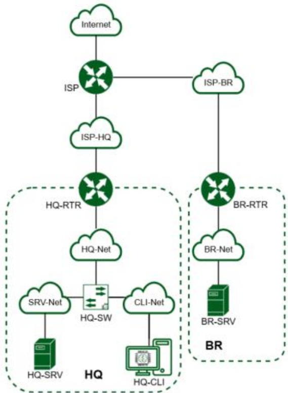
Рисунок 2. Топология сети
