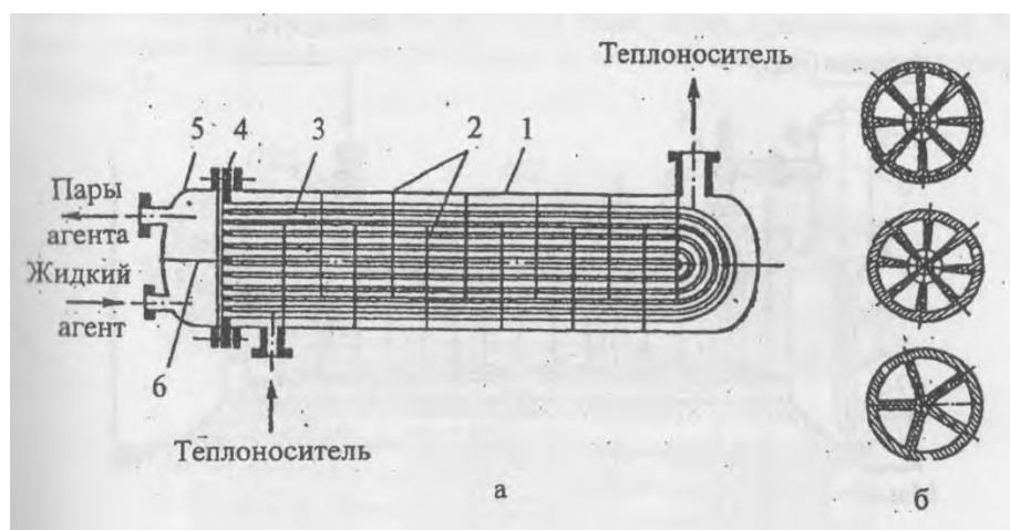
Рисунок 8. Кожухотрубный с внутритрубным кипением. Группа 1.
