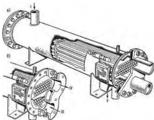
Рисунок 3. Двухходовой водяной конденсатор. Группа 1.
