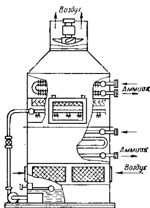
Рисунок 6. Водовоздушные конденсаторы или конденсаторы оросительного типа. Группа 3.
