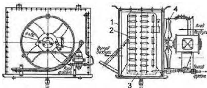
Рисунок 12. Воздушный испаритель. Группа 2б.
