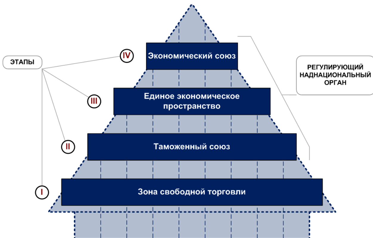
Рисунок 9 – Этапы интеграции
