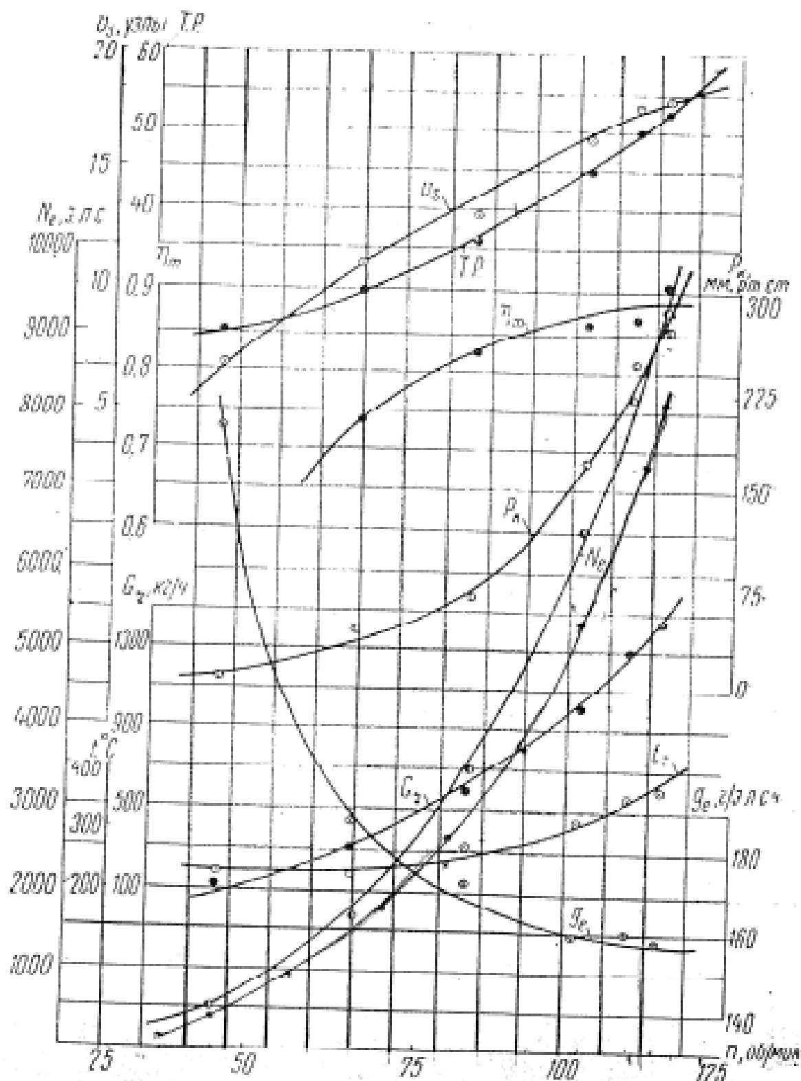
Рисунок – 1 Винтовая характеристика двигателя 8ДКРН 74/160
