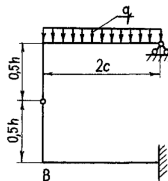
Рисунок 3.4. Расчетные схемы для типового задания №4
