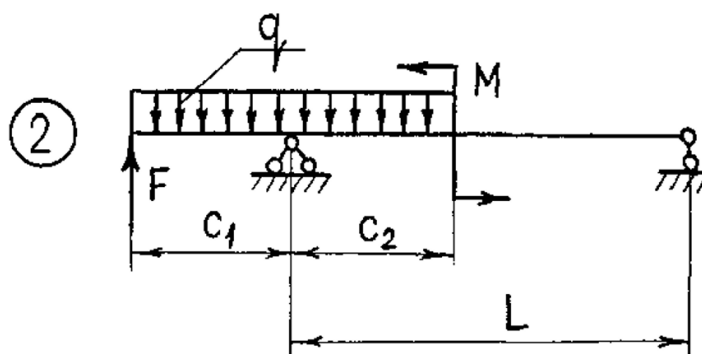
Рисунок 3.2. Расчетные схемы для типового задания №2
