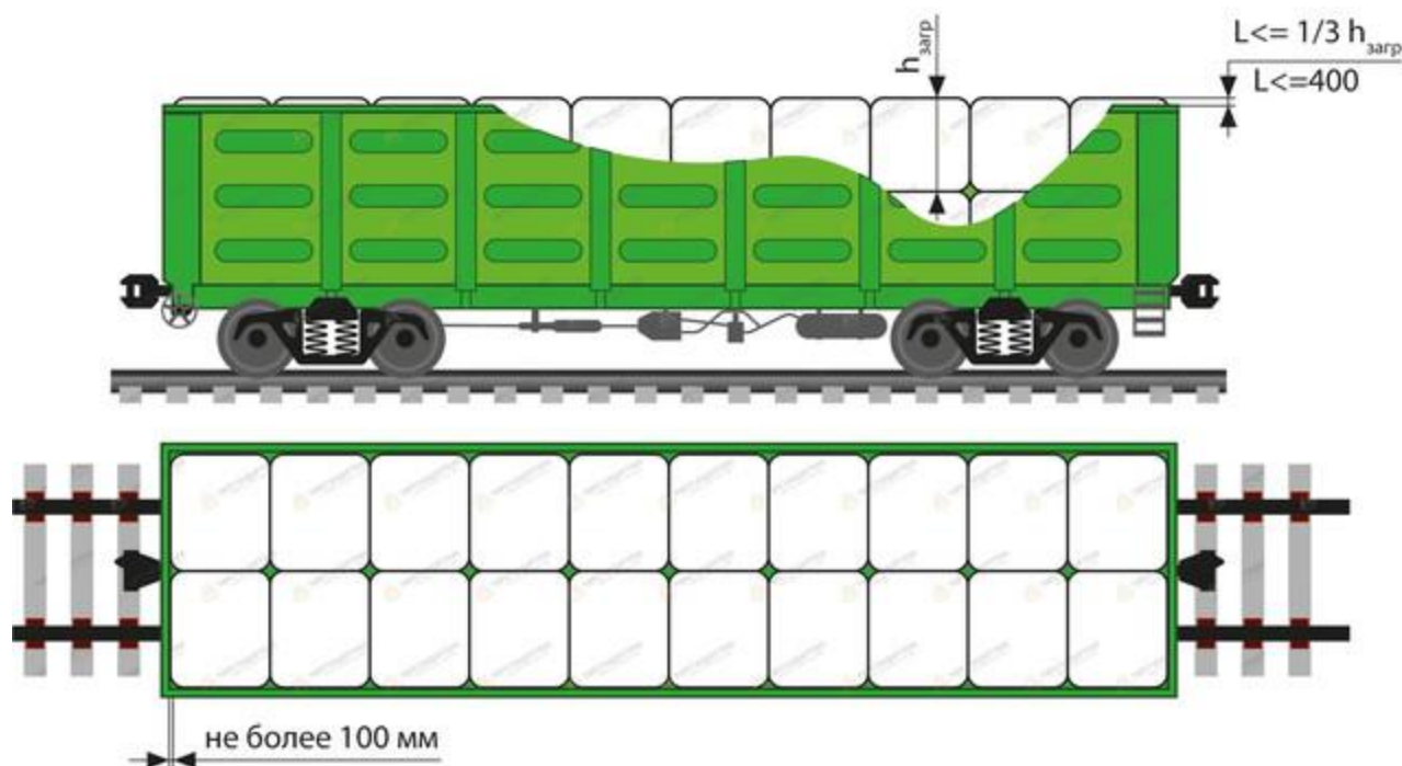
Рисунок – Пример загрузки железнодорожного вагона
