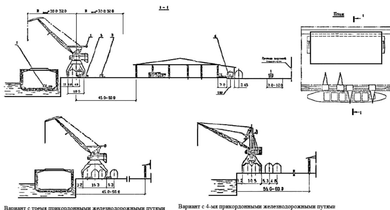
Рисунок – Примеры схем технологического процесса
