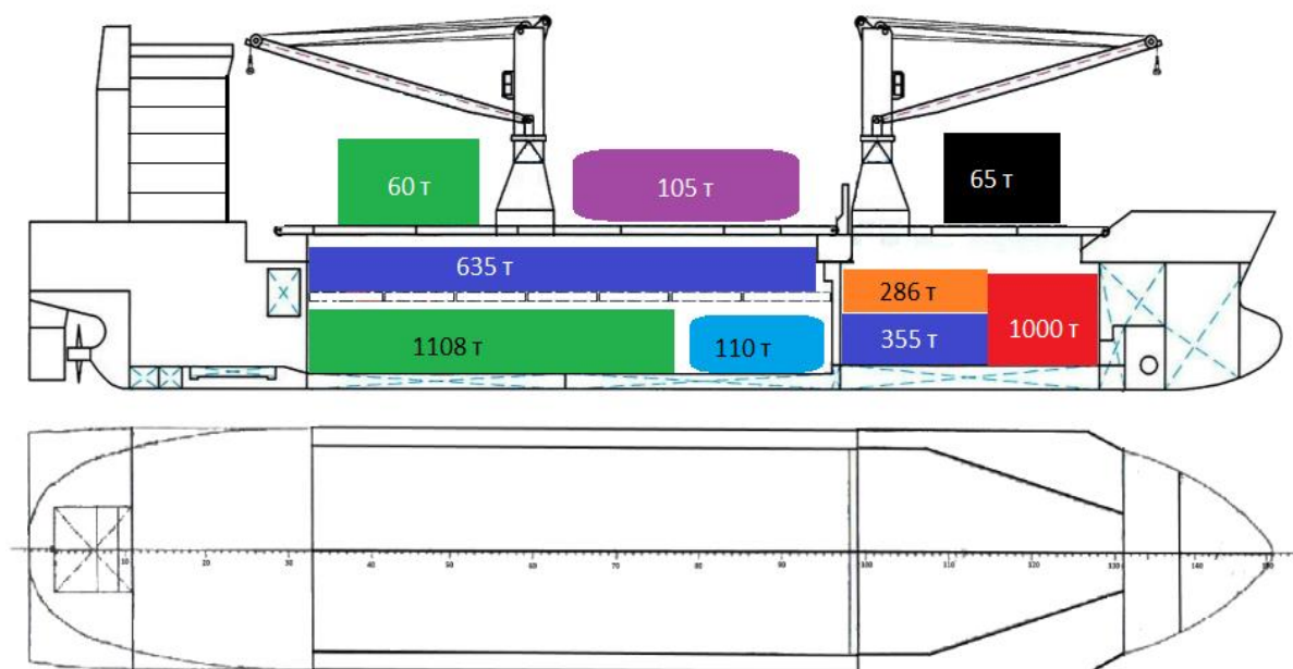
Рисунок – Пример изображения грузового плана
