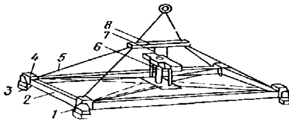
Рис.1 Автоматический приводной захват — спредер
