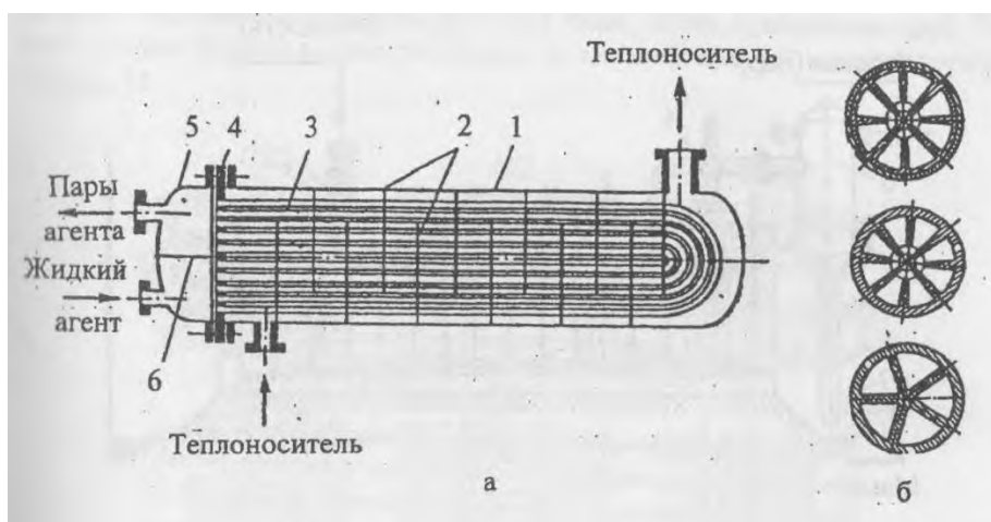
Рисунок 8. Кожухотрубчатый с внутритрубным кипением. Группа 1.
