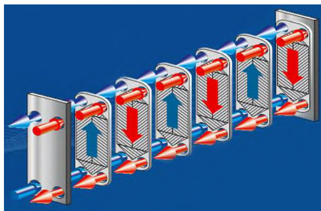
Рисунок 9. Пластины теплообменник. Группа 1.
